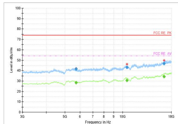
RSE-2M-CH19-3GHz-18GHz
