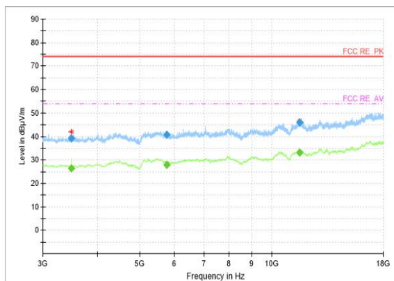
RSE-2M-CH0-3GHz-18GHz
