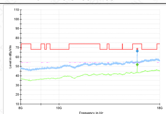
RSE-11A-CH52-8GHz-18GHz-YLD
