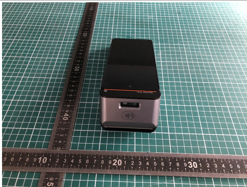
a: EUT
