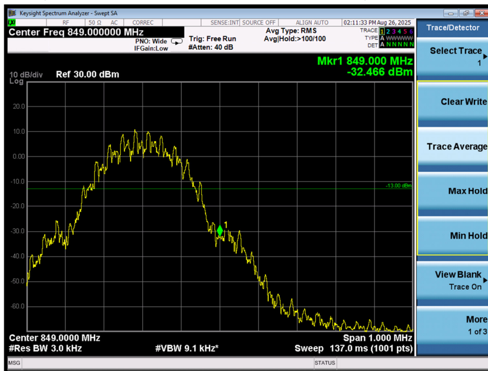
Band edge\GSM850\GPRS\H
