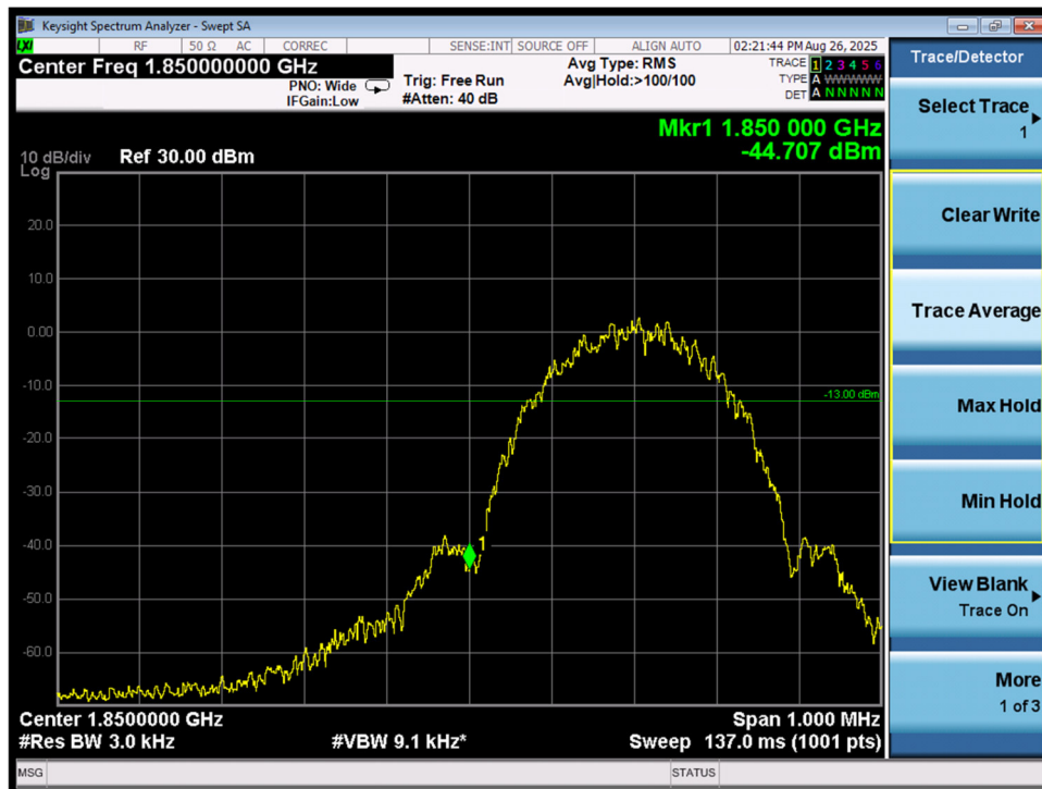
Band edge\GSM1900\EGPRS\L
