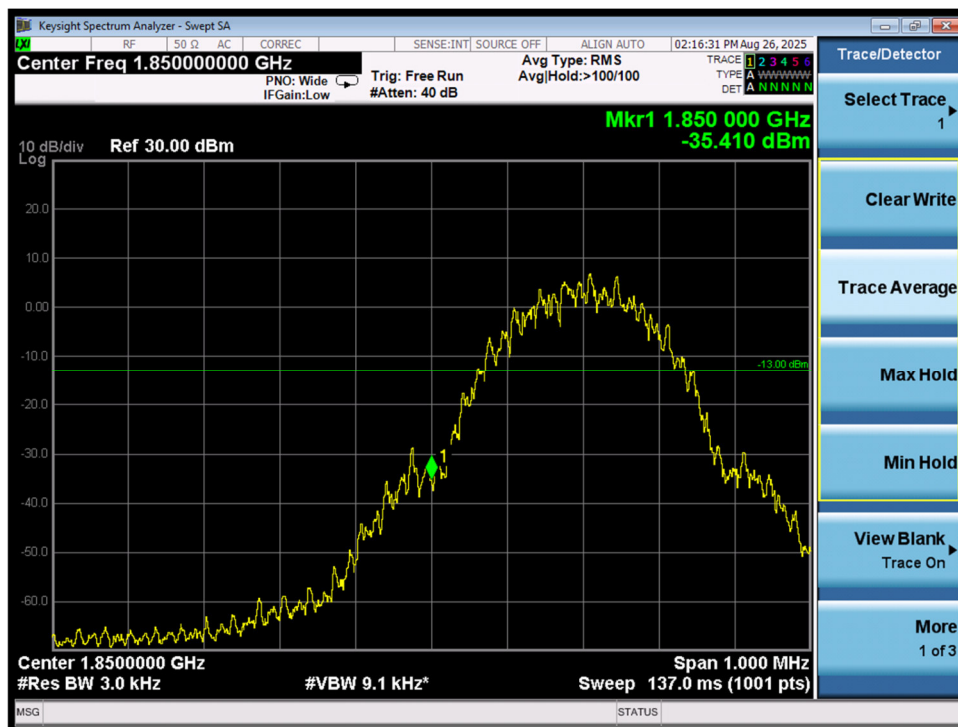
Band edge\GSM1900\GSM\L
