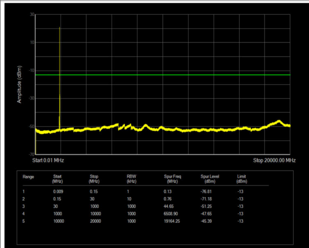
Band2 QPSK BW=15MHz Channel=19125 RB Size=1 Position=#0
