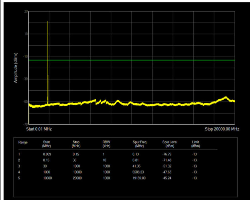
Band2 QPSK BW=20MHz Channel=18700 RB Size=1 Position=#0
