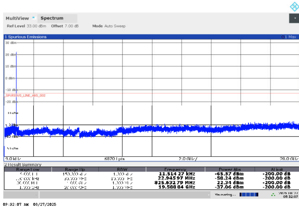
CSE\WCDMA B5\L
