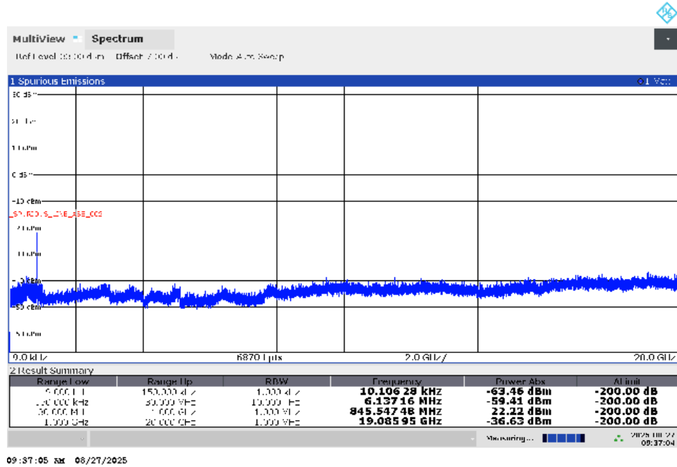
CSE\WCDMA B5\H
