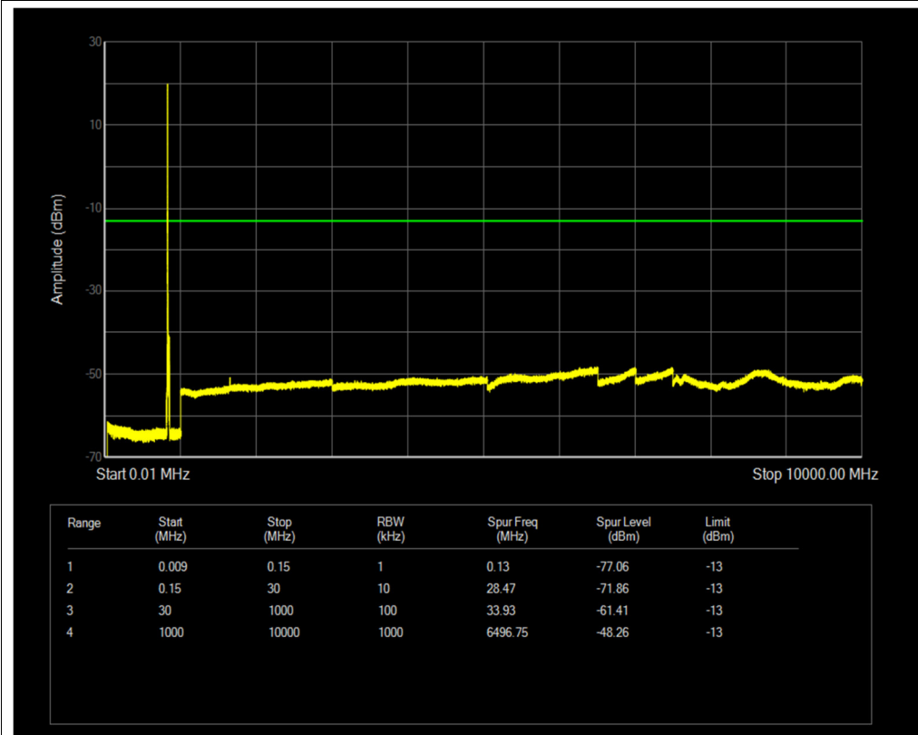
Band26(824-849) QPSK BW=15MHz Channel=26865 RB Size=1 Position=#0
