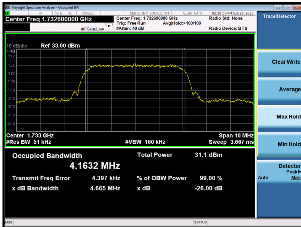
OCB\WCDMA B4\M
