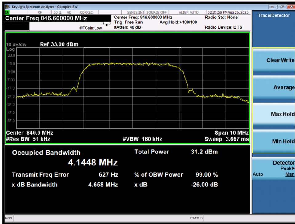
OCB\WCDMA B5\H
