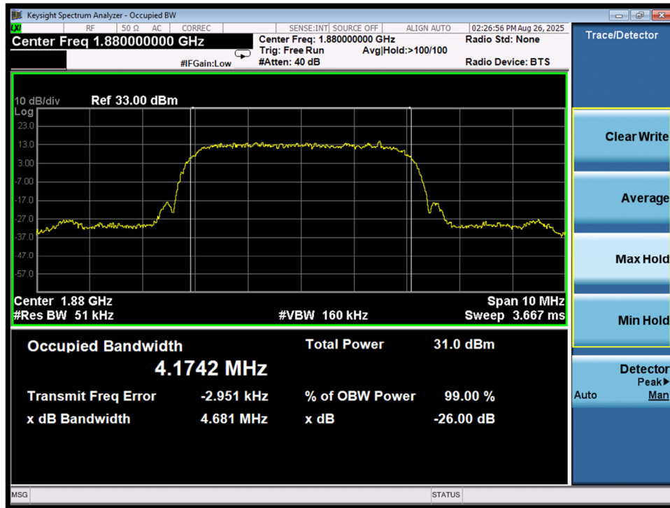
OCB\WCDMA B2\M
