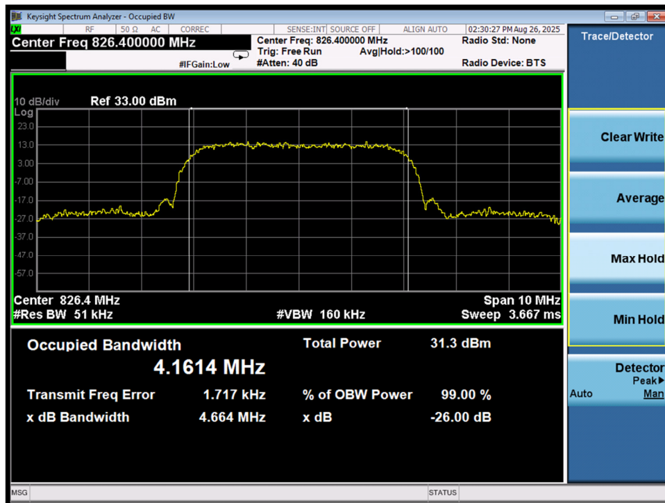
OCB\WCDMA B5\L
