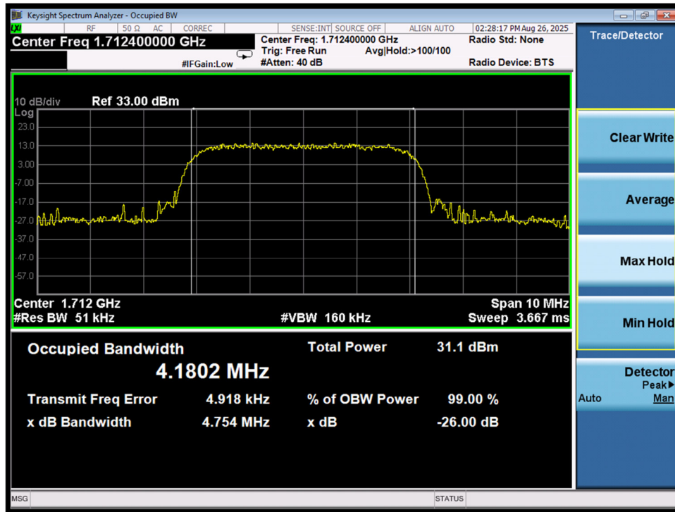
OCB\WCDMA B4\L
