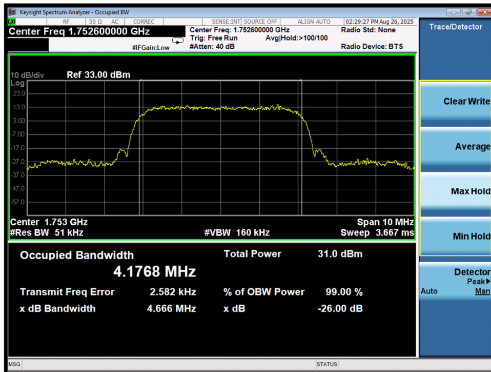
OCB\WCDMA B4\H
