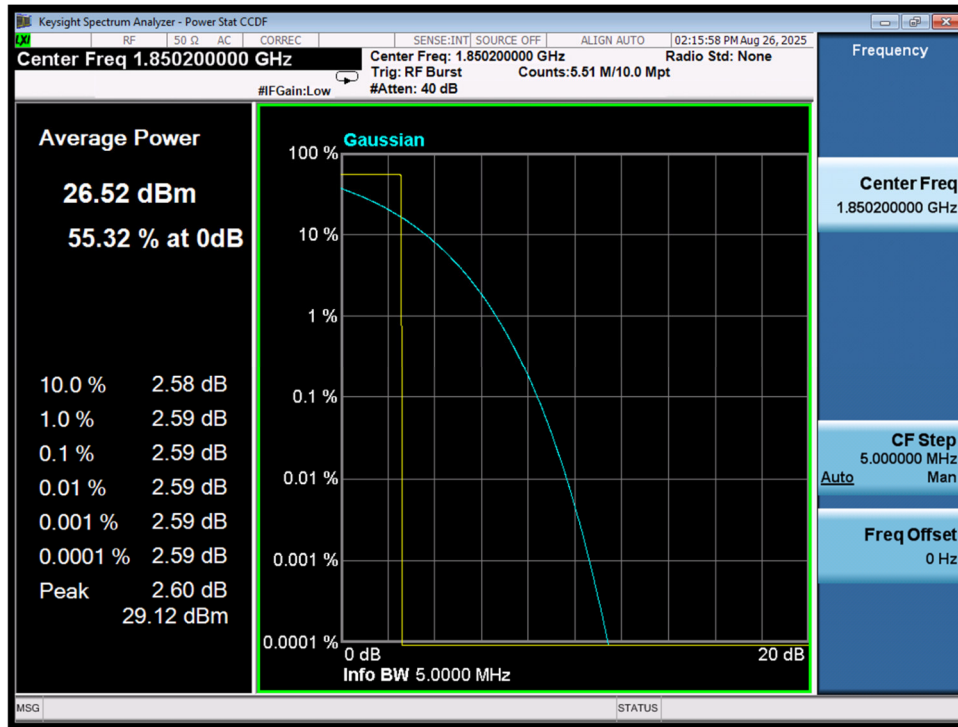
PAPR\GSM1900\GSM\L
