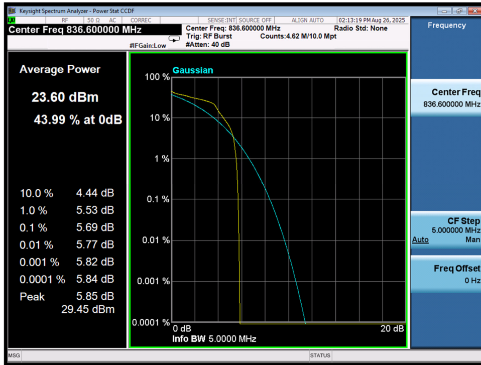
PAPR\GSM850\EGPRS\M
