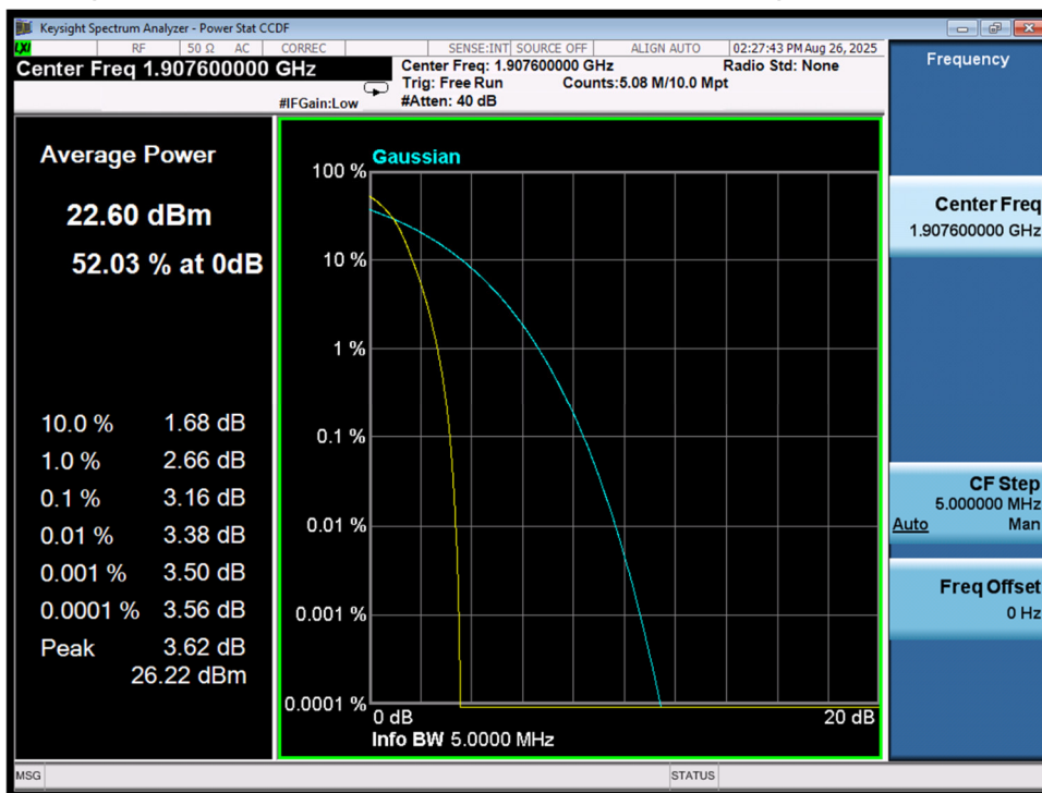
PAPRIWCDMA B2/H
