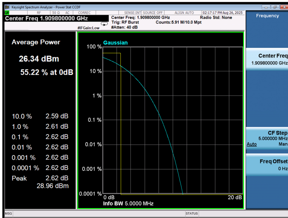
PAPR\GSM1900\GSM\H
