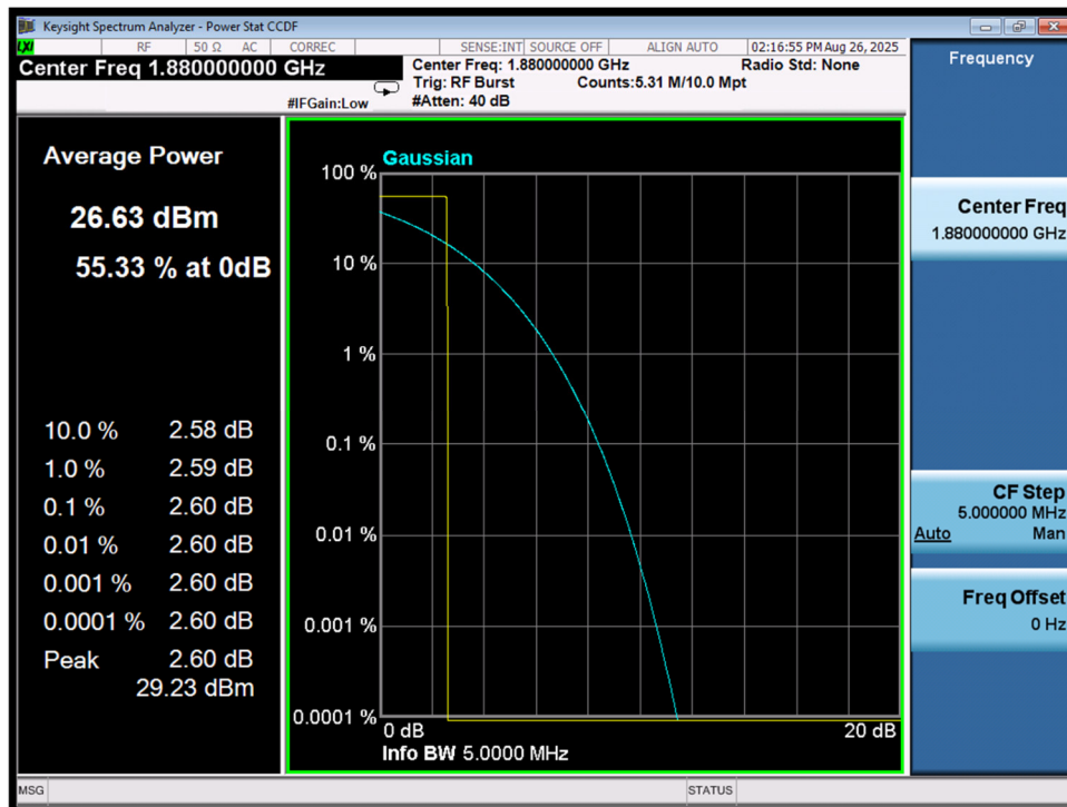
PAPR\GSM1900\GSM\M
