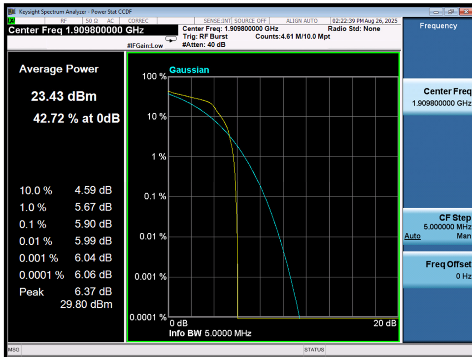
PAPR\GSM1900\EGPRS\H
