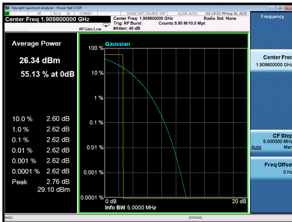
PAPR\GSM1900\GPRS\H
