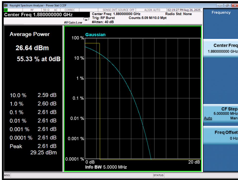
PAPR\GSM1900\GPRS\M
