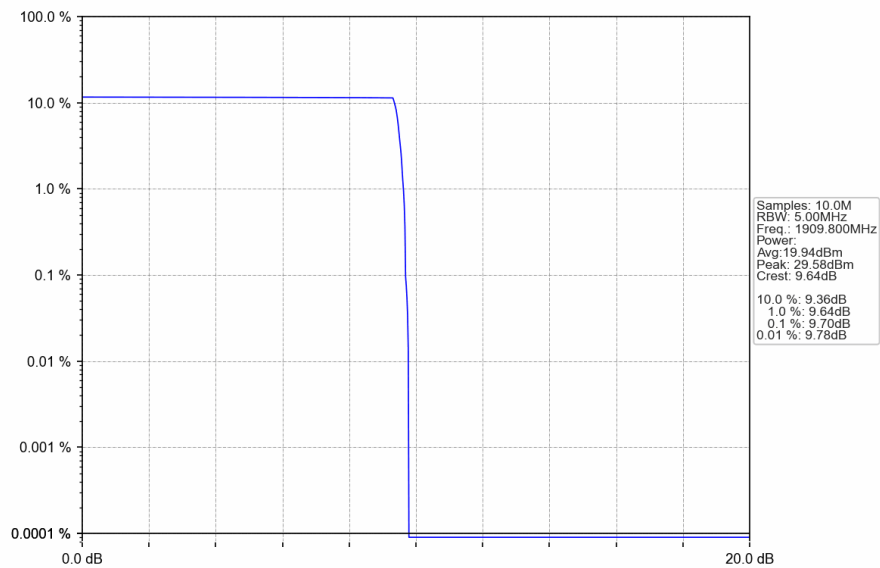
PCS1900_GSM_HCH_1909.8MHz_GSM_NTNV
