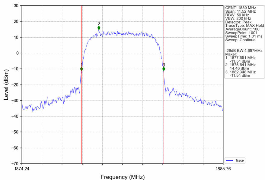
Band2_HSUPA_MCH_1880MHz_Subtest 1_NTNV
