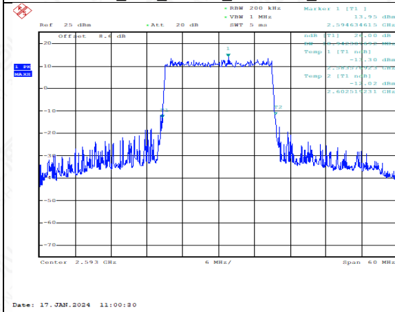
TDD41_Mid_20MHz_2593MHz_QPSK
