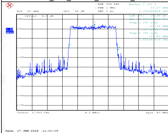
TDD41_Mid_20MHz_2593MHz_QPSK
