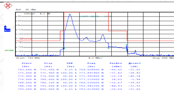
FDD13LowRange_10MHz_QPSK_1RB_LowRange
