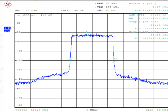
FDD26(PART 22)_MidRange_3MHz_836.5MHz _QPSK
