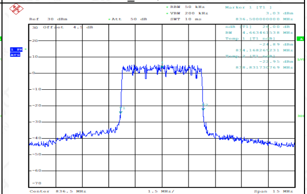
FDD26(PART 22)_MidRange_5MHz_836.5MHz _16QAM
