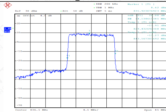
FDD26(PART 22)_MidRange_15MHz_836.5MHz_QPSK
