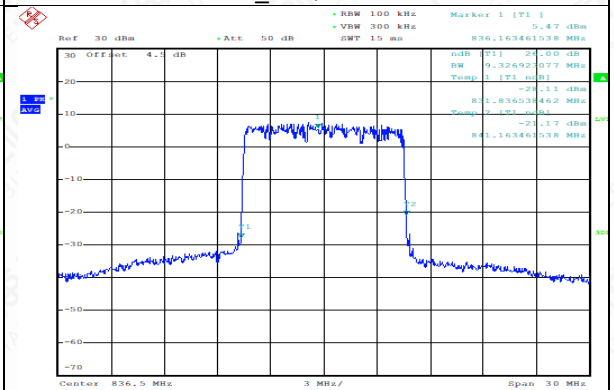
FDD26(PART 22)_MidRange_10MHz_836.5MHz _16QAM
