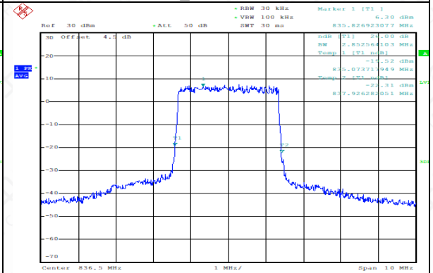
FDD26(PART 22)_MidRange_3MHz_836.5MHz _16QAM
