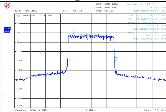
FDD26(PART 22)_MidRange_10MHz_836.5MHz _QPSK
