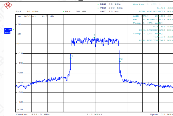
FDD26(PART 22)_MidRange_5MHz_836.5MHz _QPSK
