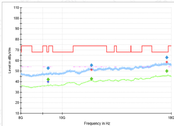
RSE-11AC(40M)-CH159-8GHz-18GHz
