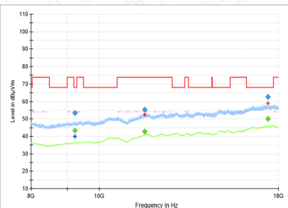
RSE-11AC(80M)-CH155-8GHz-18GHz
