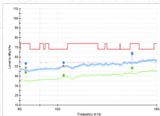
RSE-11N(20M)-CH36-8GHz-18GHz
