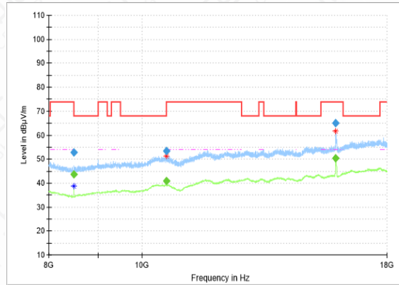
RSE-11N(40M)-CH62-8GHz-18GHz
