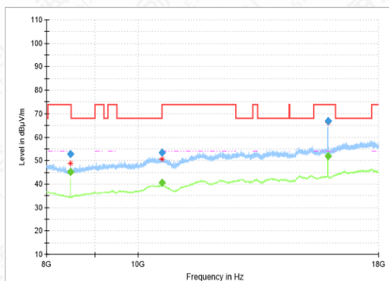
RSE-11N(20M)-CH60-8GHz-18GHz
