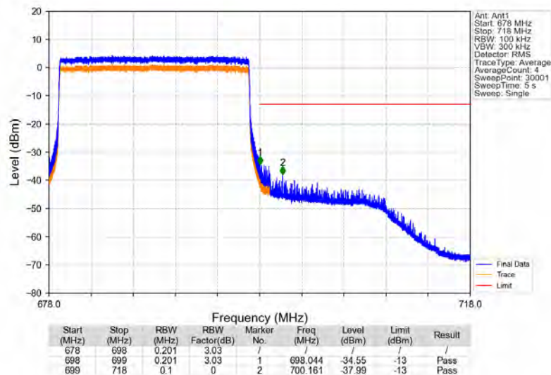
Band71_20MHz_16QAM_HCH_688MHz_RB_100_0_NTNV
