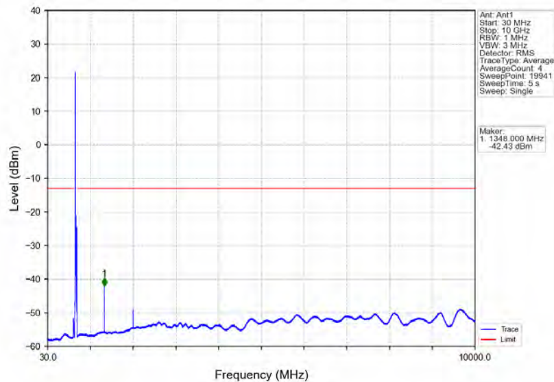
Band71_20MHz_16QAM_HCH_688MHz_RB_1_0_NTNV
