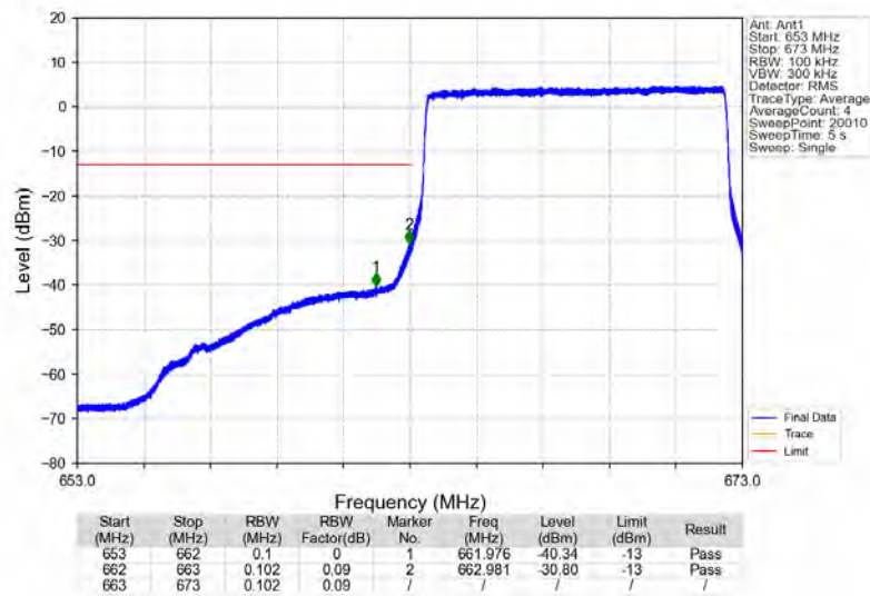
Band71_10MHz_QPSK_LCH_668MHz_RB_50_0_NTNV
