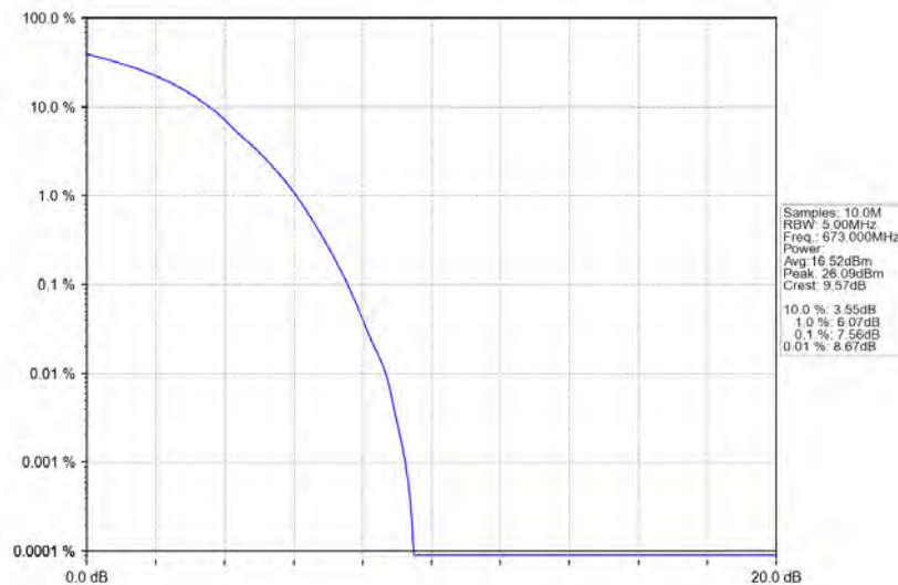
Band71_20MHz_16QAM_LCH_673MHz_RB_100_0_NTNV
