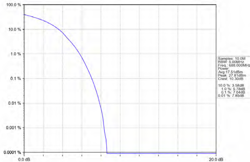
Band71_20MHz_QPSK_HCH_688MHz_RB_100_0_NTNV
