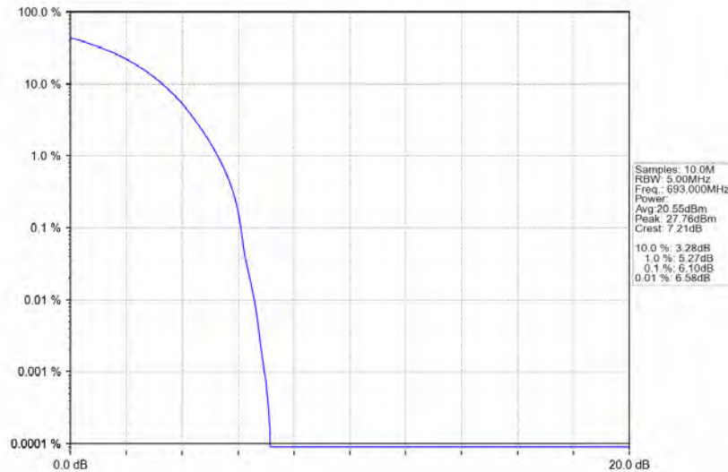
Band71_10MHz_QPSK_HCH_693MHz_RB_50_0_NTNV
