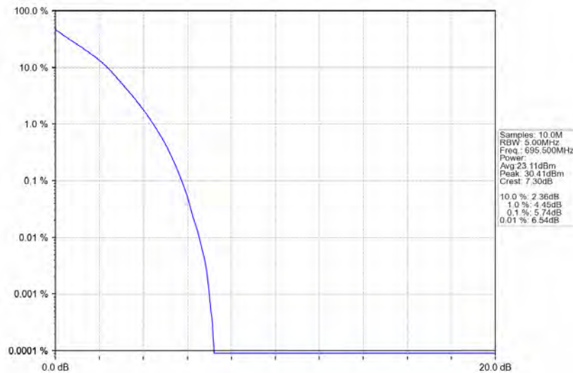
Band71_5MHz_QPSK_HCH_695.5MHz_RB_25_0_NTNV
