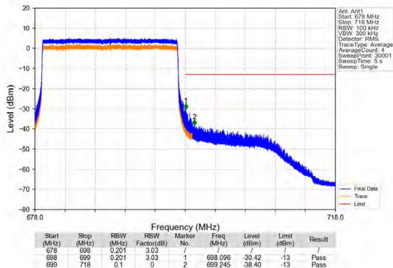
Band71_20MHz_QPSK_HCH_688MHz_RB_100_0_NTNV
