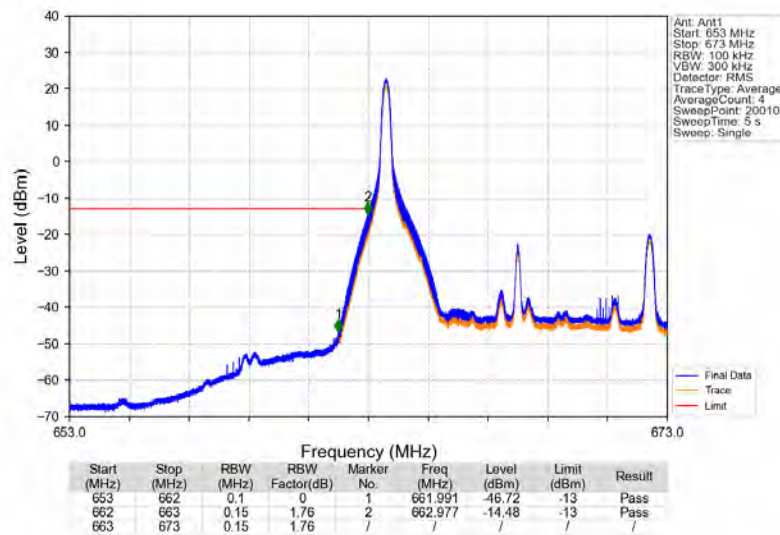
Band71 10MHz 16QAM LCH 668MHz RB 1 0 NTNV
