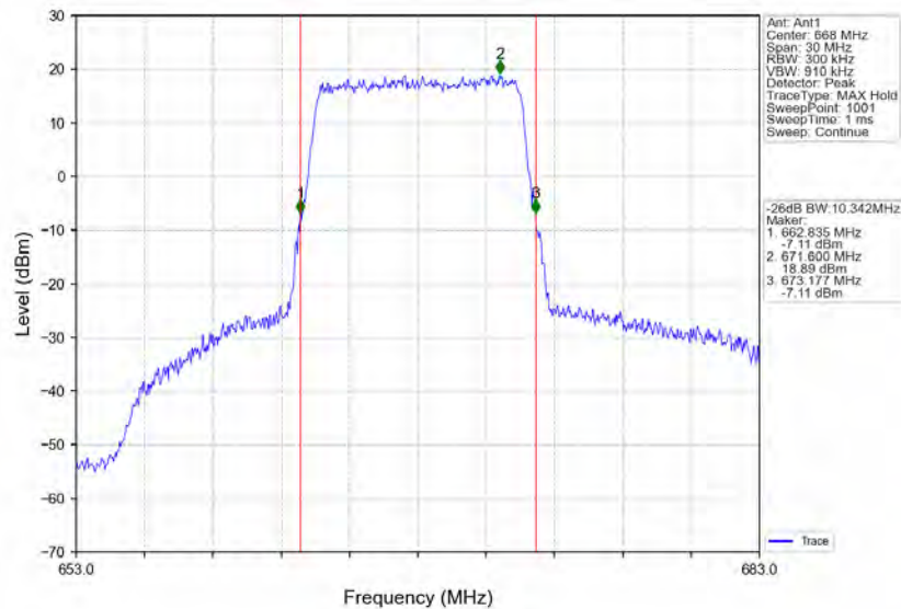
Band71_10MHz_QPSK_LCH_668MHz_RB_50_0_NTNV
