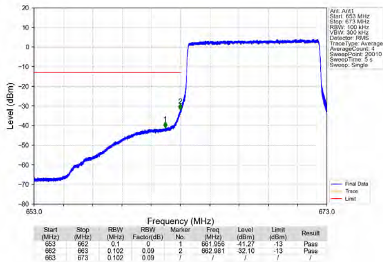
Band71_10MHz_16QAM_LCH_668MHz_RB_50_0_NTNV
