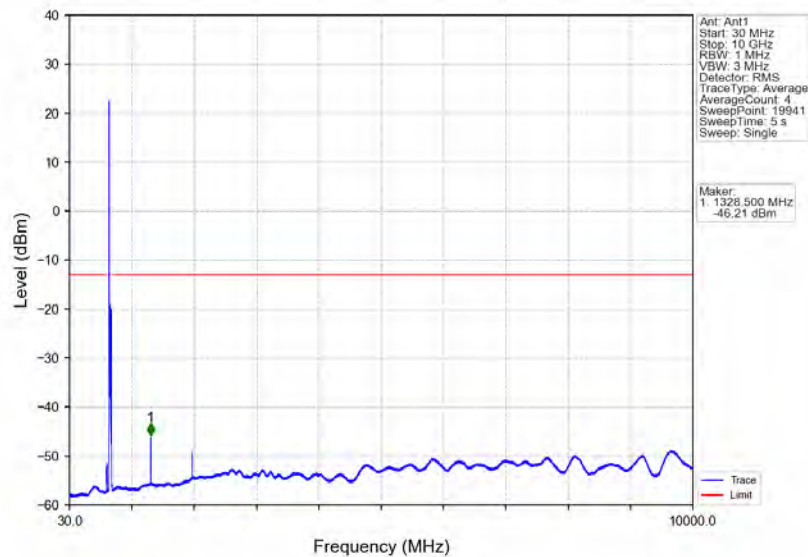
Band71 20MHz 16QAM LCH 673MHz RB 100 0 NTNV
