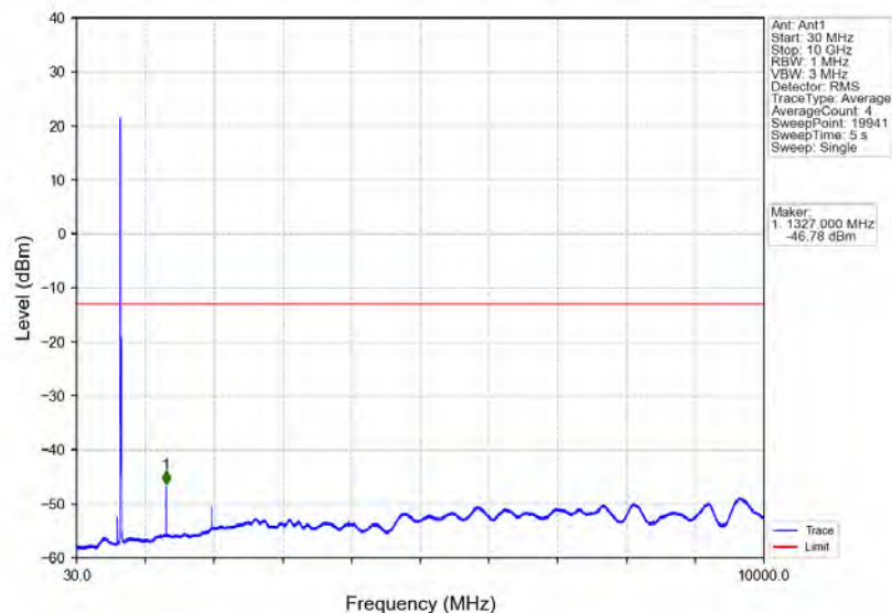
Band71 10MHz 64QAM LCH 668MHz RB 1 0 NTNV
