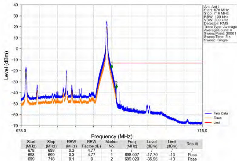
Band71_20MHz_16QAM_HCH_688MHz_RB_1_99_NTNV
