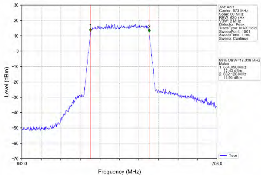
Band71 20MHz 64QAM LCH 673MHz RB 100 0 NTNV
