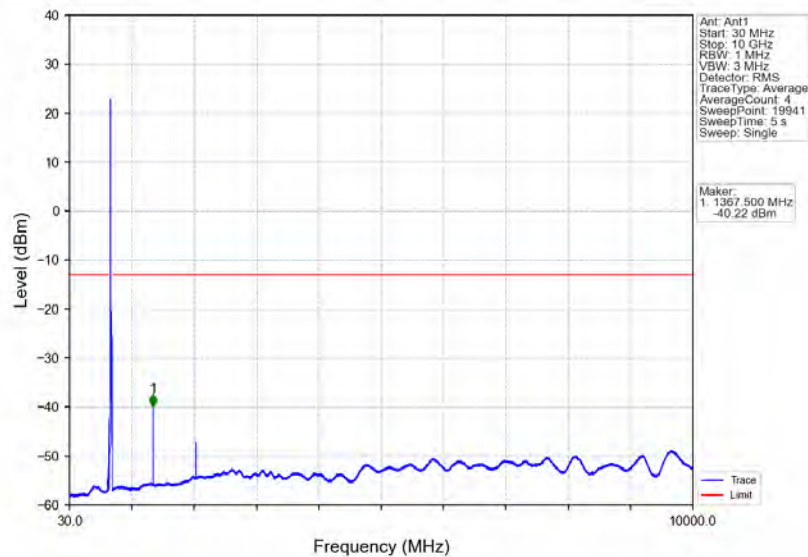
Band71_15MHz_QPSK_HCH_690.5MHz_RB_1_74_NTNV
