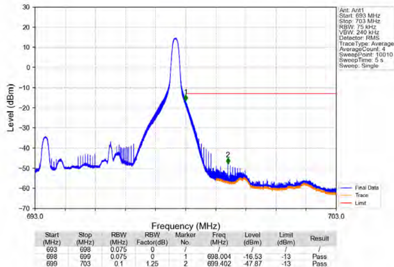
Band71_5MHz_QPSK_HCH_695.5MHz_RB_1_24_NTNV
