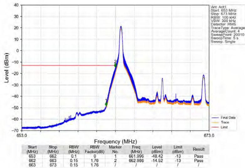
Band71 10MHz 64QAM LCH 668MHz RB 1 0 NTNV
