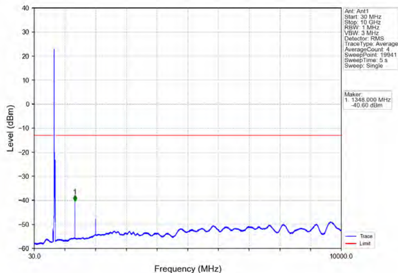
Band71_20MHz_QPSK_MCH_683MHz_RB_1_0_NTNV
