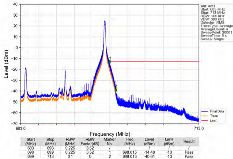
Band71_15MHz_QPSK_HCH_690.5MHz_RB_1_74_NTNV
