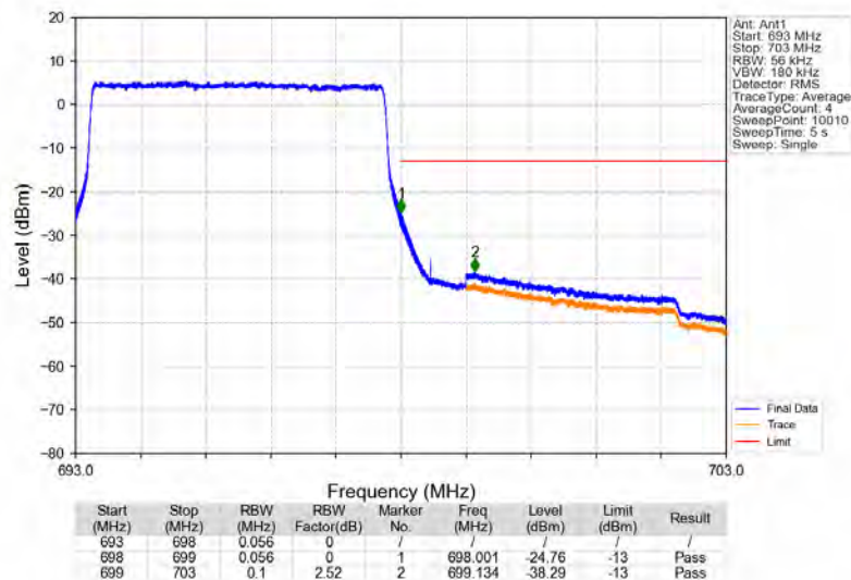
Band71_5MHz_QPSK_HCH_695.5MHz_RB_25_0_NTNV
