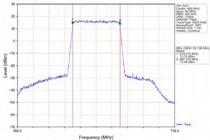
Band71 20MHz 64QAM HCH 688MHz RB 100 0 NTNV
