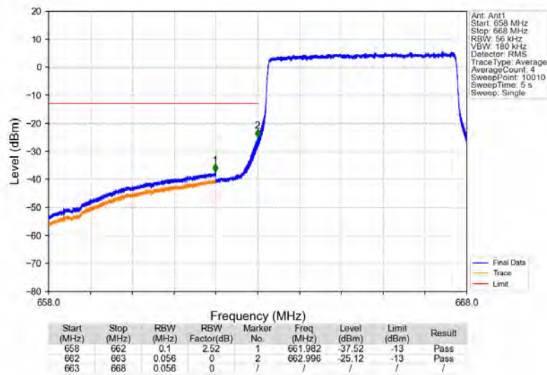
Band71_5MHz_QPSK_LCH_665.5MHz_RB_25_0_NTNV
