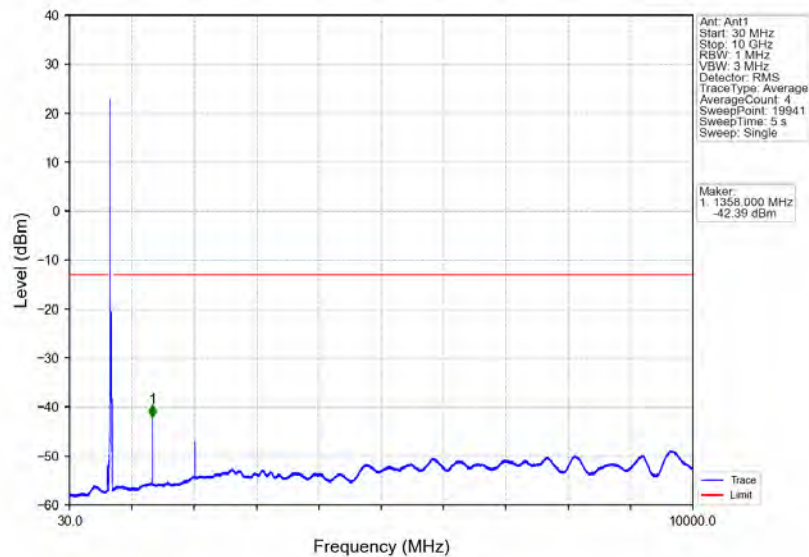
Band71_20MHz_QPSK_HCH_688MHz_RB_1_99_NTNV
