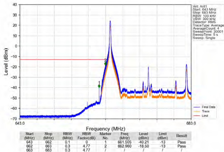
Band71 20MHz 64QAM LCH 673MHz RB 1 0 NTNV
