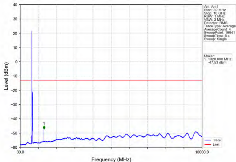
Band71 20MHz 64QAM LCH 673MHz RB 1 0 NTNV
