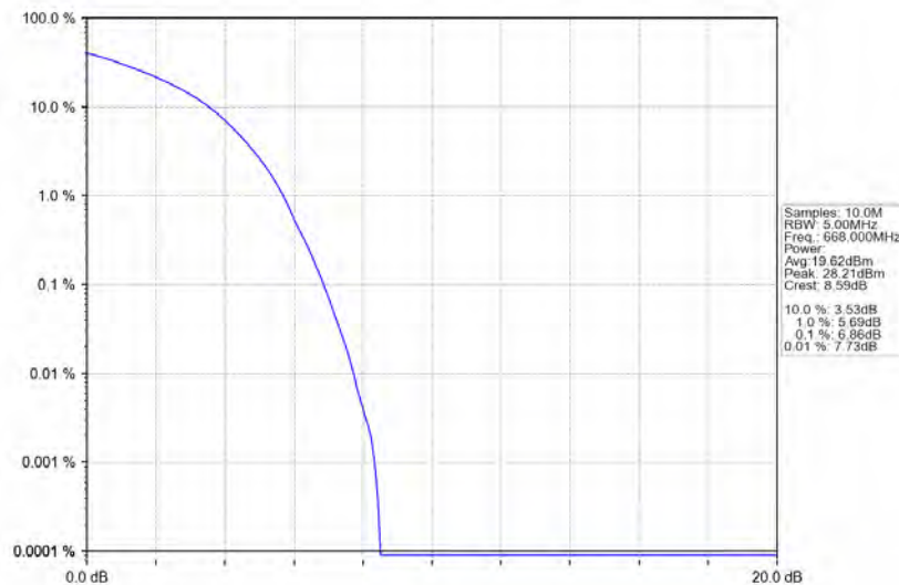
Band71_10MHz_16QAM_LCH_668MHz_RB_50_0_NTNV
