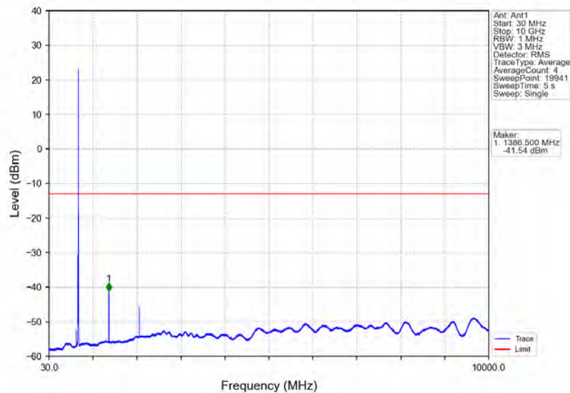
Band71_5MHz_QPSK_HCH_695.5MHz_RB_1_24_NTNV
