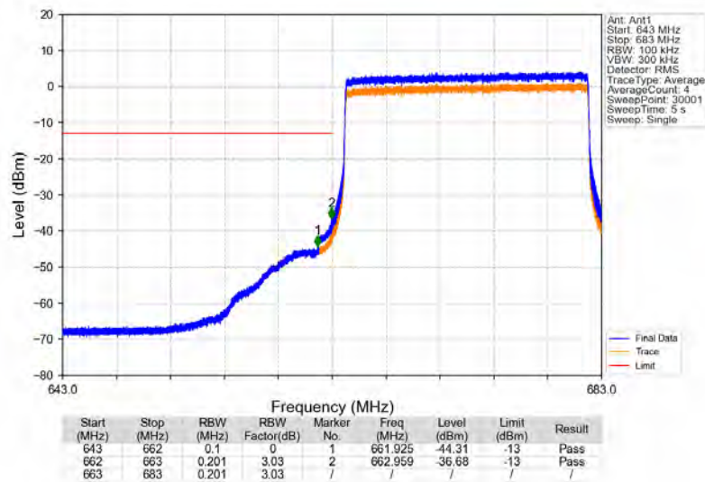
Band71 20MHz 16QAM LCH 673MHz RB 100 0 NTNV
