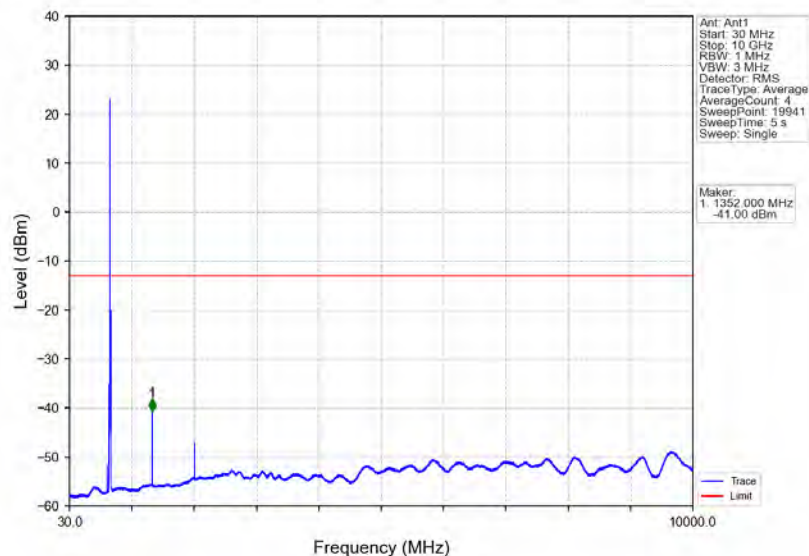
Band71_10MHz_QPSK_MCH_680.5MHz_RB_1_0_NTNV
