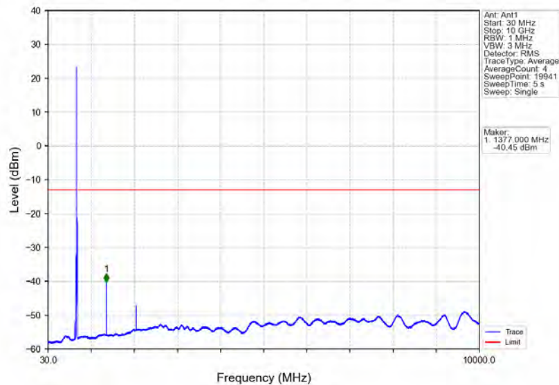
Band71_10MHz_QPSK_HCH_693MHz_RB_1_49_NTNV
