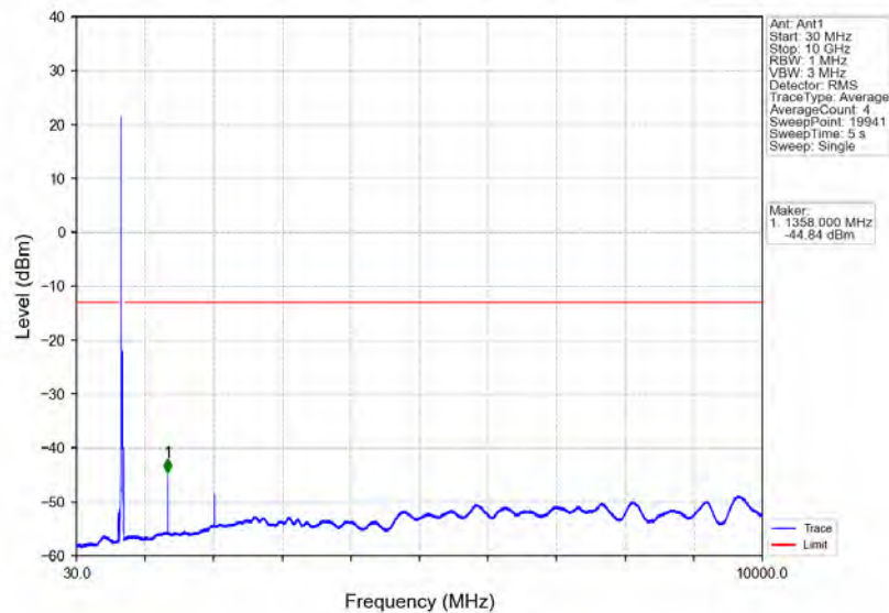
Band71_20MHz_64QAM_HCH_688MHz_RB_1_99_NTNV
