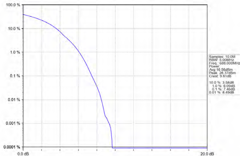
Band71_20MHz_16QAM_HCH_688MHz_RB_100_0_NTNV
