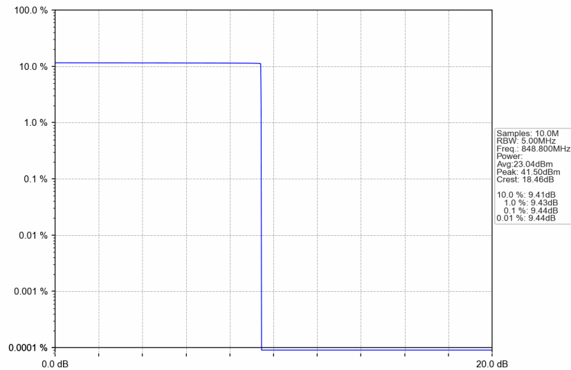
GSM850_GSM_HCH_848.8MHz_GSM_NTNV
