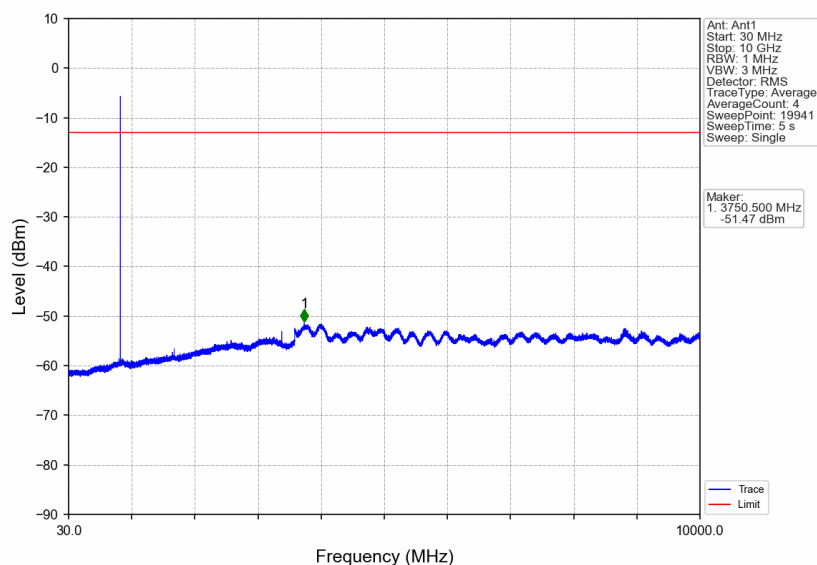
GSM850_EGPRS_HCH_848.8MHz_1 TX Slot_NTNV
