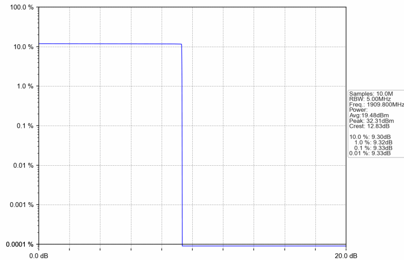
PCS1900_GSM_HCH_1909.8MHz_GSM_NTNV
