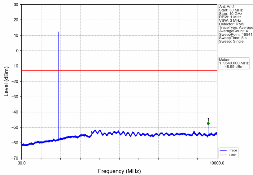
PCS1900_GSM_HCH_1909.8MHz_GSM_NTNV
