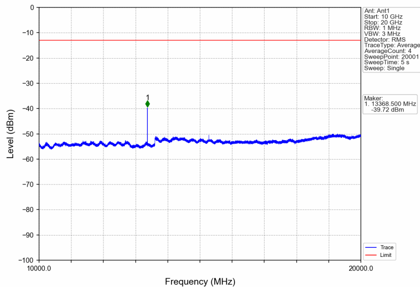
PCS1900_GSM_HCH_1909.8MHz_GSM_NTNV
