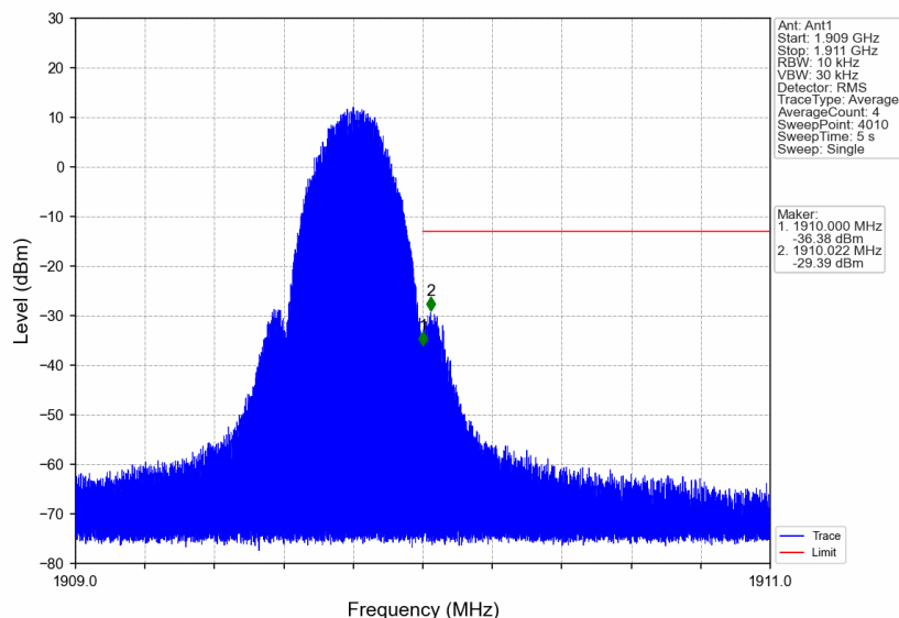
PCS1900_EGPRS_HCH_1909.8MHz_1 TX Slot_NTNV
