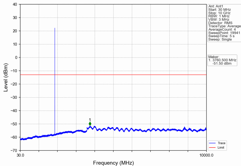
PCS1900_GSM_MCH_1880MHz_GSM_NTNV
