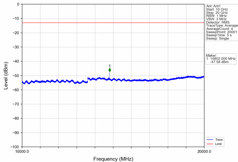
PCS1900_GSM_MCH_1880MHz_GSM_NTNV
