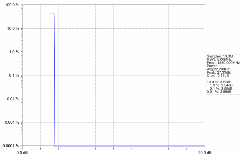
PCS1900_GPRS_MCH_1880MHz_4 TX Slots_NTNV
