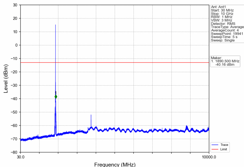
Band2_HSUPA_MCH_1880MHz_Subtest 1_NTNV
