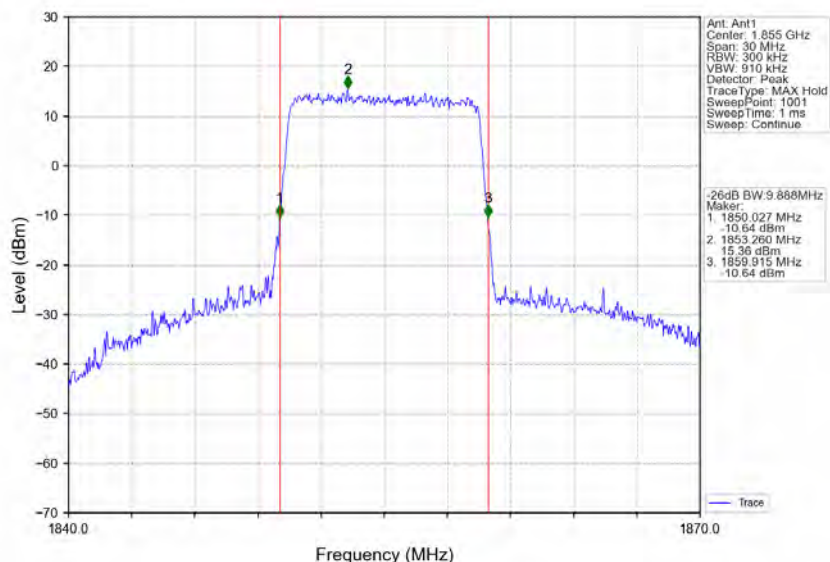
Band2_10MHz_64QAM_LCH_1855MHz_RB_50_0_NTNV
