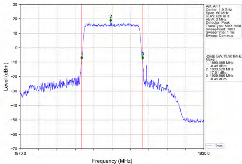
Band2_20MHz_QPSK_HCH_1900MHz_RB_100_0_NTNV
