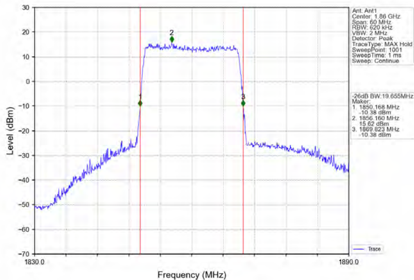
Band2_20MHz_64QAM_LCH_1860MHz_RB_100_0_NTNV
