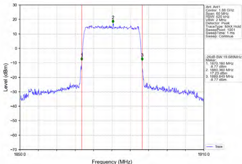
Band2_20MHz_16QAM_MCH_1880MHz_RB_100_0_NTNV
