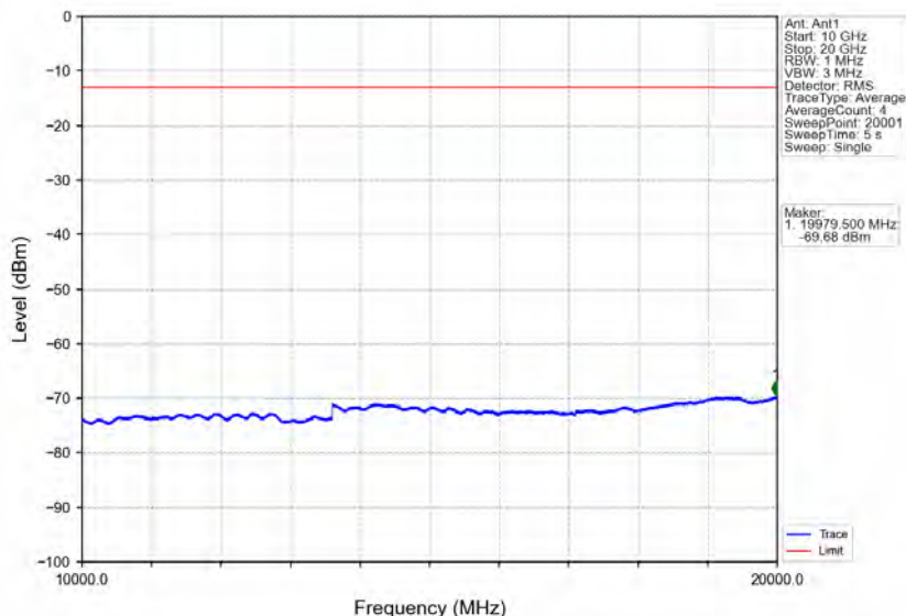
Band2_10MHz_QPSK_MCH_1880MHz_RB_1_0_NTNV
