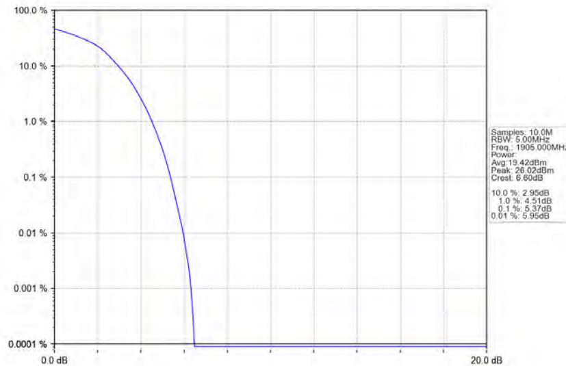
Band2_10MHz_QPSK_HCH_1905MHz_RB_50_0_NTNV
