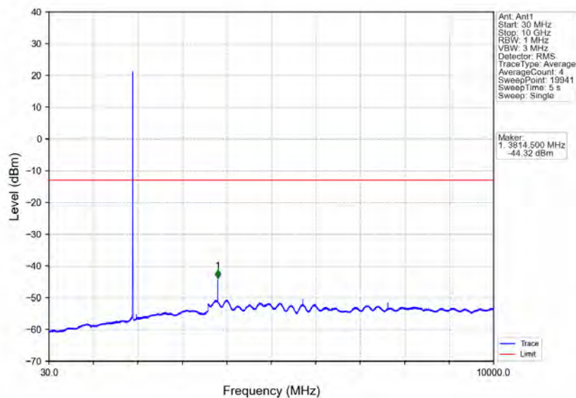
Band2_3MHz_QPSK_HCH_1908.5MHz_RB_1_0_NTNV
