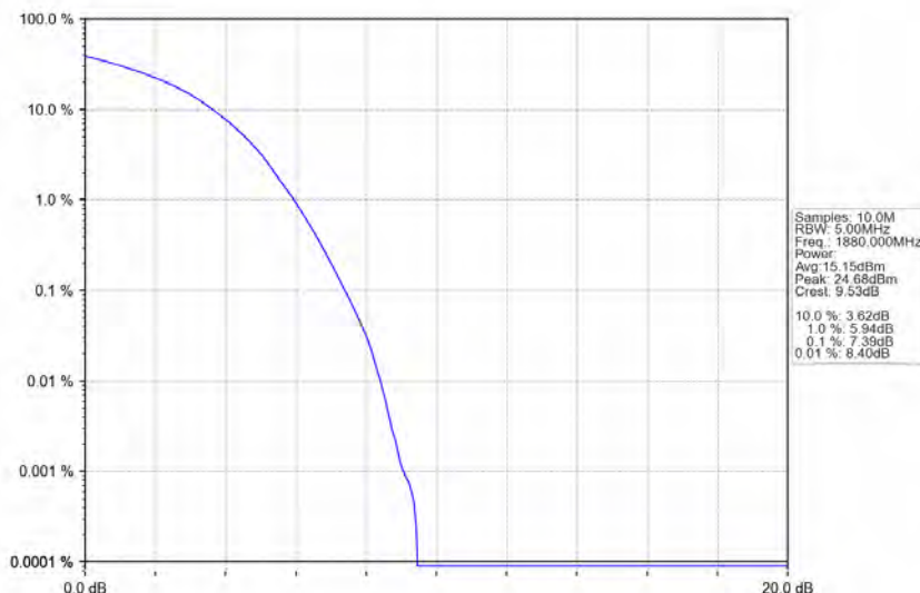
Band2_20MHz_16QAM_MCH_1880MHz_RB_100_0_NTNV
