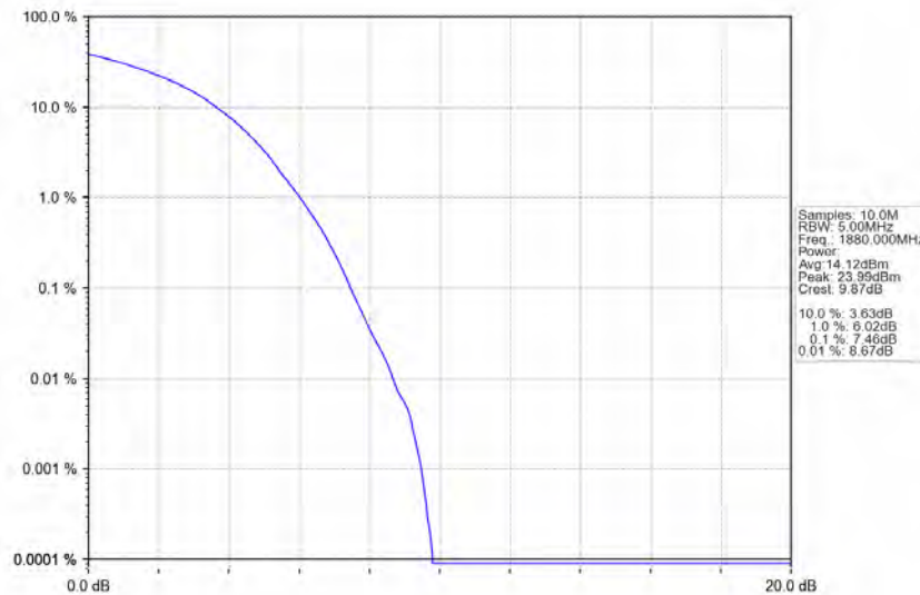
Band2_20MHz_64QAM_MCH_1880MHz_RB_100_0_NTNV
