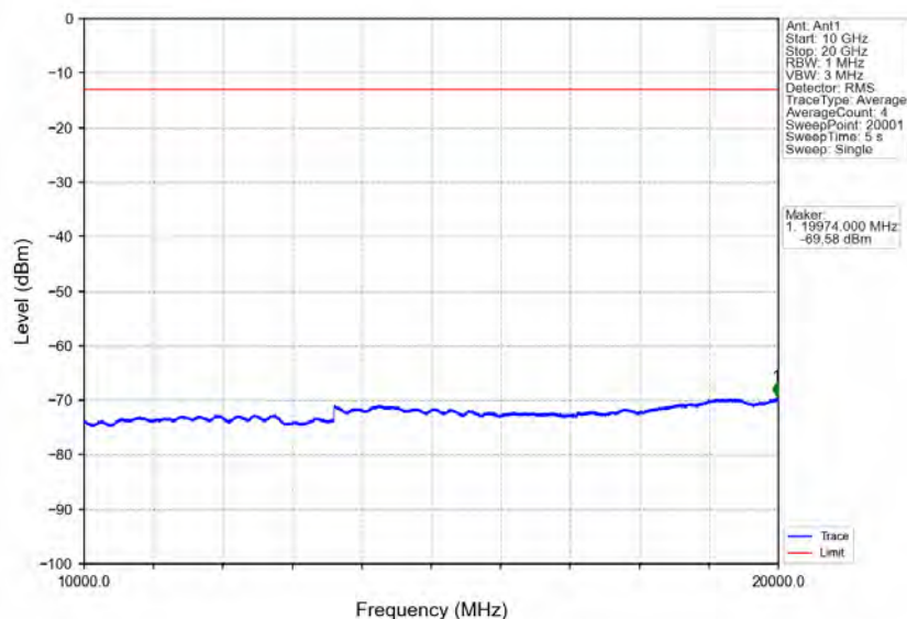
Band2_10MHz_QPSK_LCH_1855MHz_RB_50_0_NTNV
