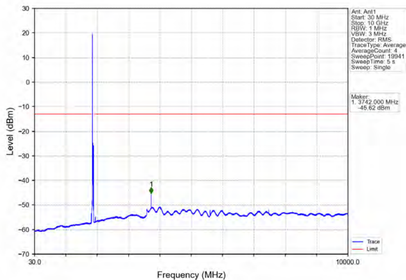
Band2_20MHz_64QAM_MCH_1880MHz_RB_1_0_NTNV
