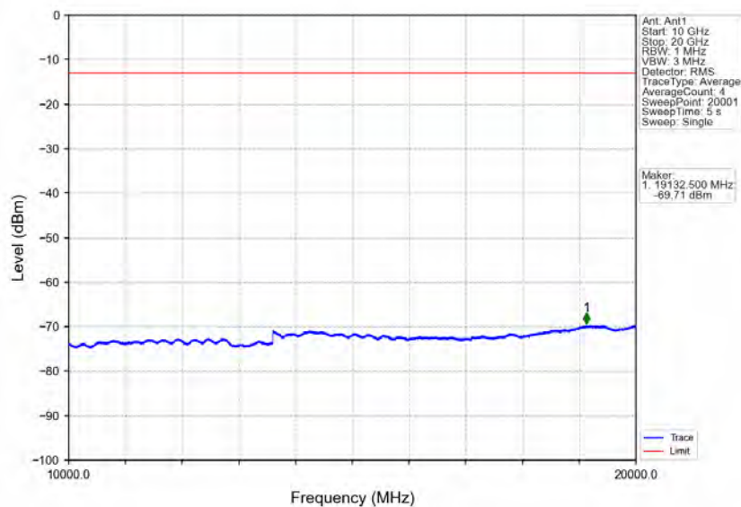
Band2_20MHz_QPSK_MCH_1880MHz_RB_1_0_NTNV
