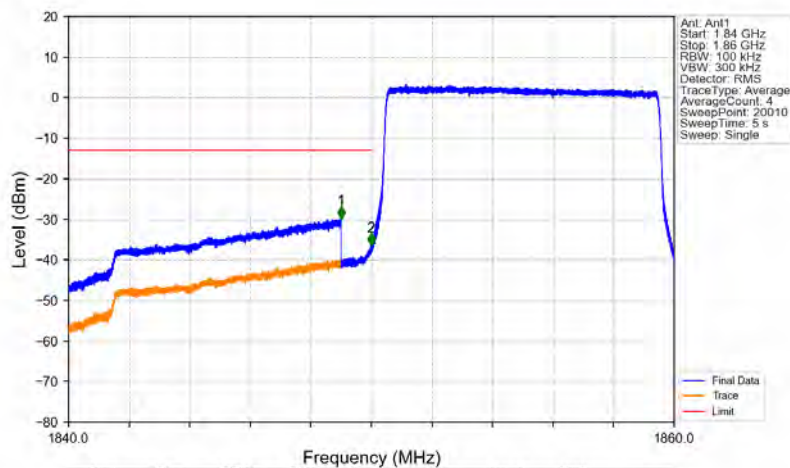
Band2_10MHz_QPSK_LCH_1855MHz_RB_50_0_NTNV
