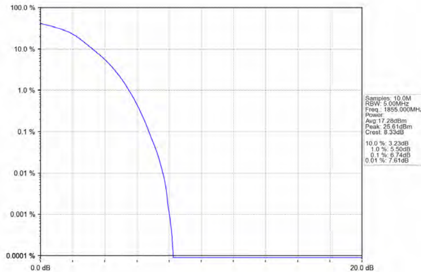
Band2_10MHz_64QAM_LCH_1855MHz_RB_50_0_NTNV
