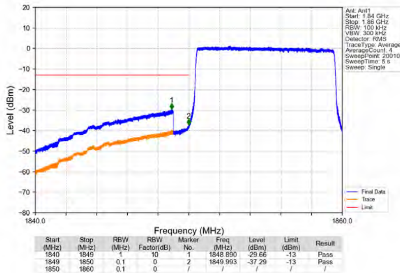
Band2_10MHz_64QAM_LCH_1855MHz_RB_50_0_NTNV
