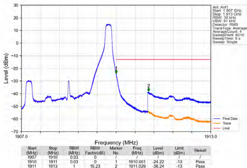
Band2_3MHz_QPSK_HCH_1908.5MHz_RB_1_14_NTNV
