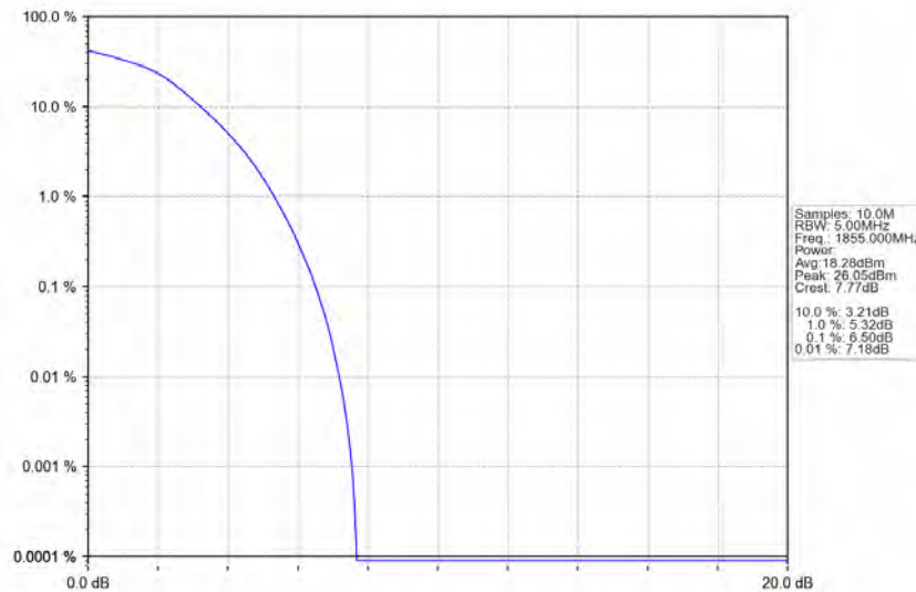
Band2_10MHz_16QAM_LCH_1855MHz_RB_50_0_NTNV
