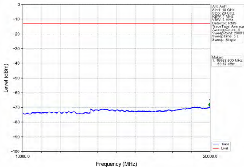
Band2_20MHz_QPSK_LCH_1860MHz_RB_100_0_NTNV
