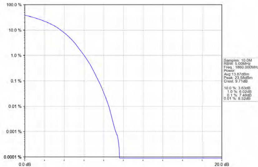
Band2_20MHz_64QAM_LCH_1860MHz_RB_100_0_NTNV
