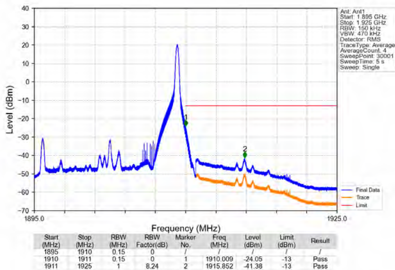
Band2_15MHz_16QAM_HCH_1902.5MHz_RB_1_74_NTNV
