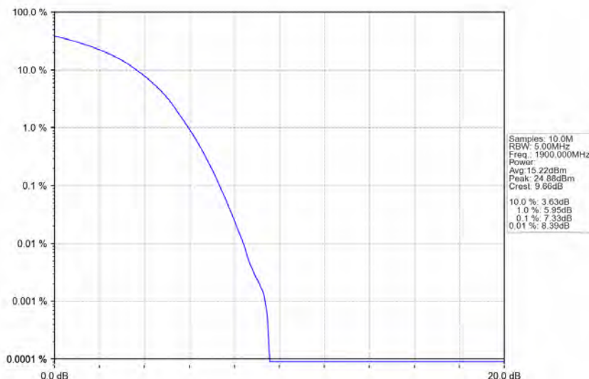
Band2_20MHz_16QAM_HCH_1900MHz_RB_100_0_NTNV
