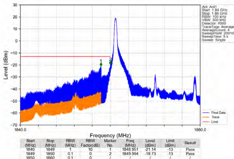
Band2_10MHz_16QAM_LCH_1855MHz_RB_1_0_NTNV
