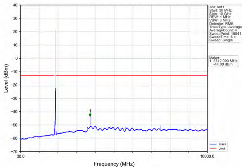
Band2_20MHz_QPSK_MCH_1880MHz_RB_1_0_NTNV
