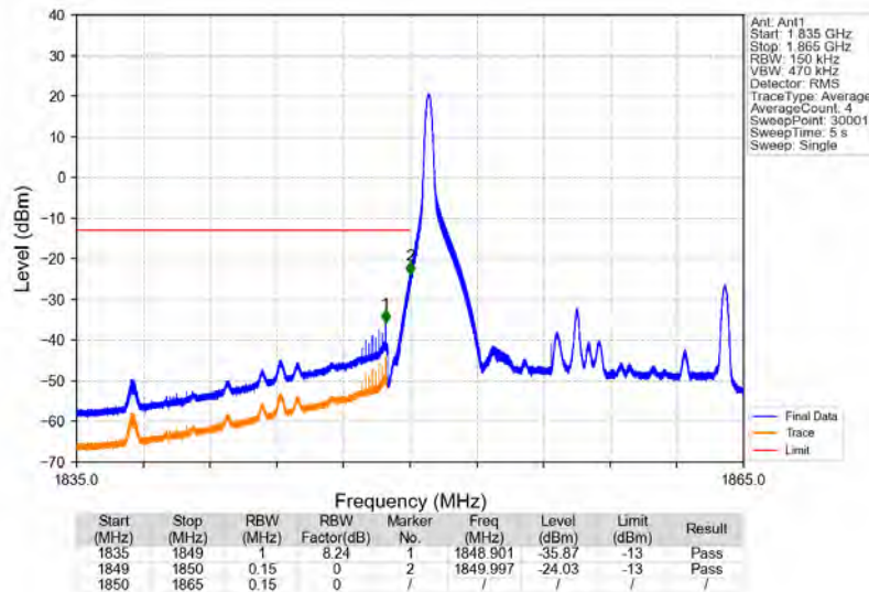
Band2_15MHz_QPSK_LCH_1857.5MHz_RB_1_0_NTNV
