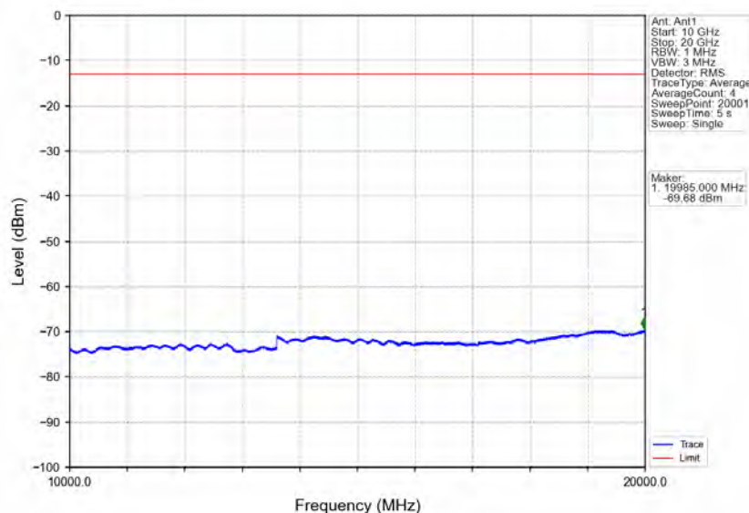
Band2_20MHz_16QAM_LCH_1860MHz_RB_100_0_NTNV
