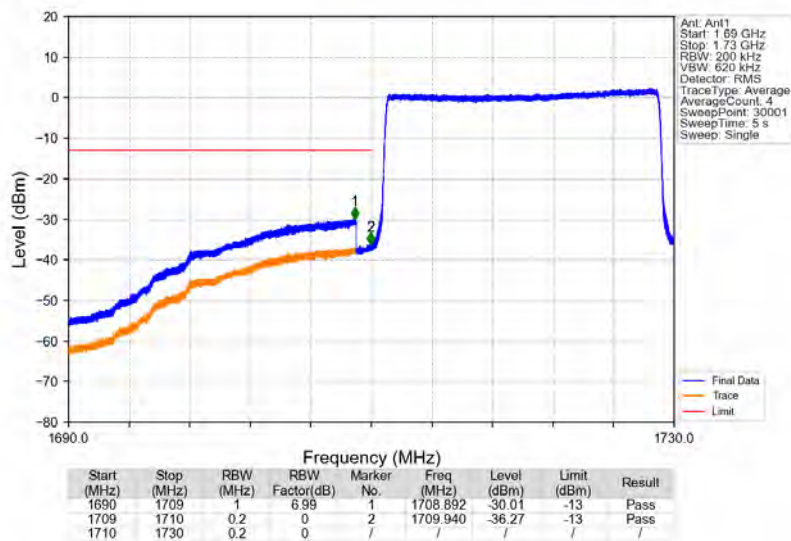
Band4_20MHz_16QAM_LCH_1720MHz_RB_100_0_NTNV
