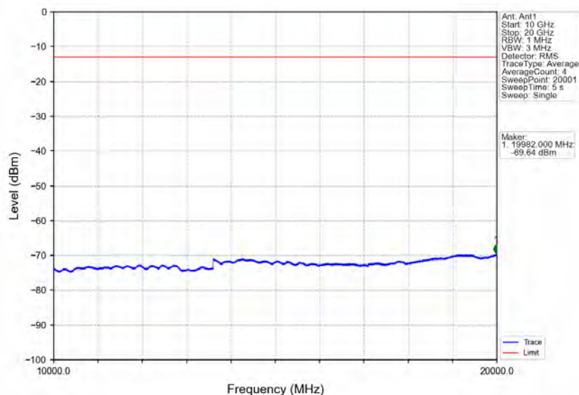
Band4_20MHz_16QAM_LCH_1720MHz_RB_100_0_NTNV
