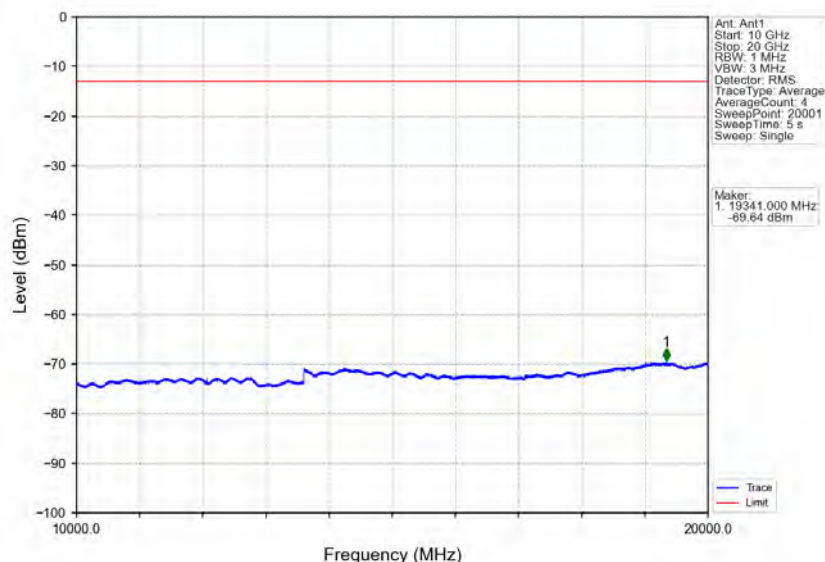
Band4_20MHz_QPSK_MCH_1732.5MHz_RB_1_0_NTNV
