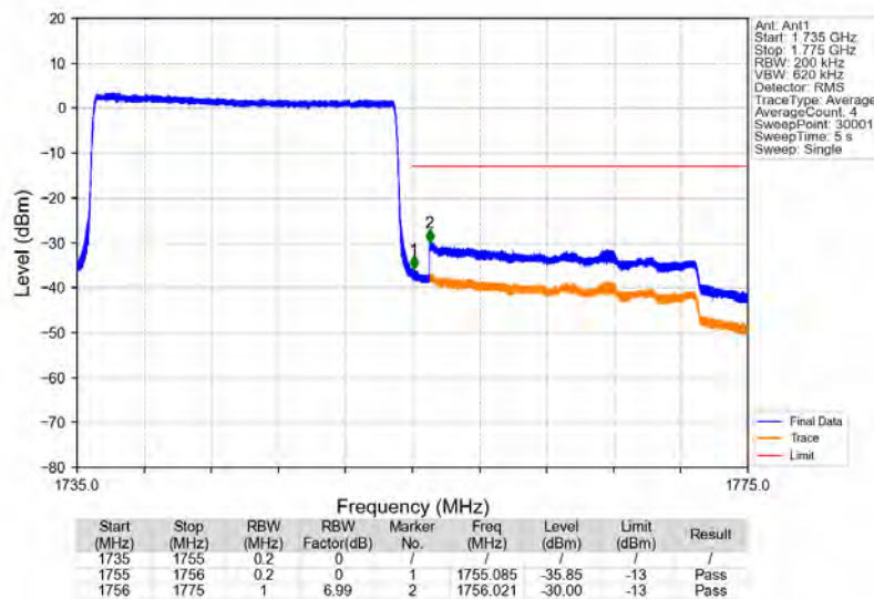
Band4_20MHz_QPSK_HCH_1745MHz_RB_100_0_NTNV
