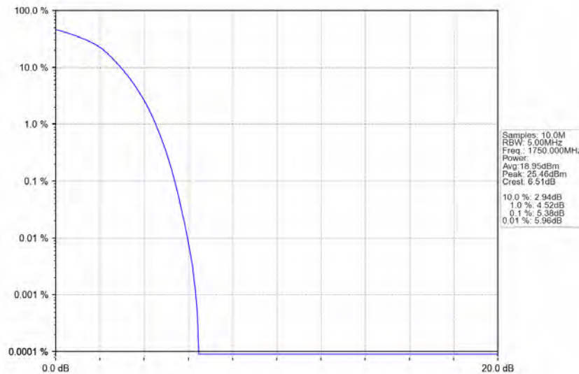
Band4_10MHz_QPSK_HCH_1750MHz_RB_50_0_NTNV
