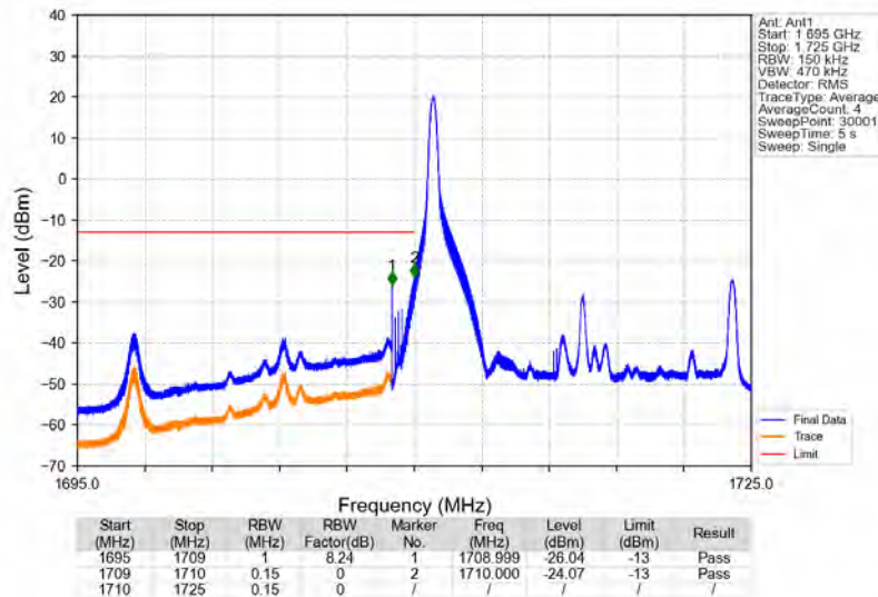
Band4_15MHz_QPSK_LCH_1717.5MHz_RB_1_0_NTNV
