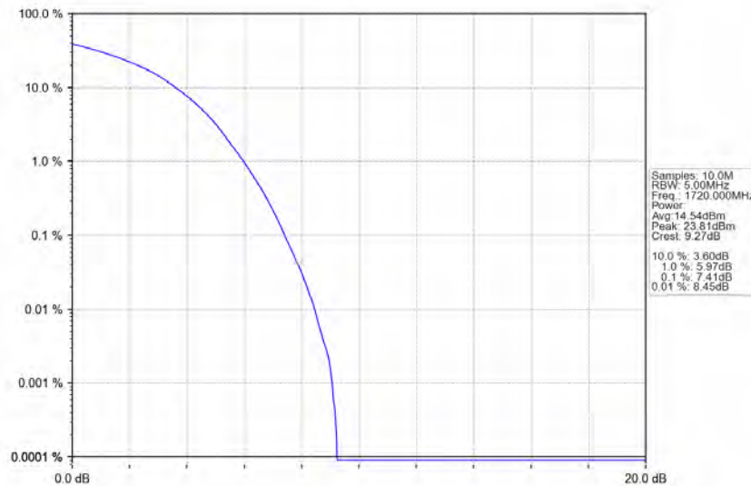
Band4_20MHz_16QAM_LCH_1720MHz_RB_100_0_NTNV
