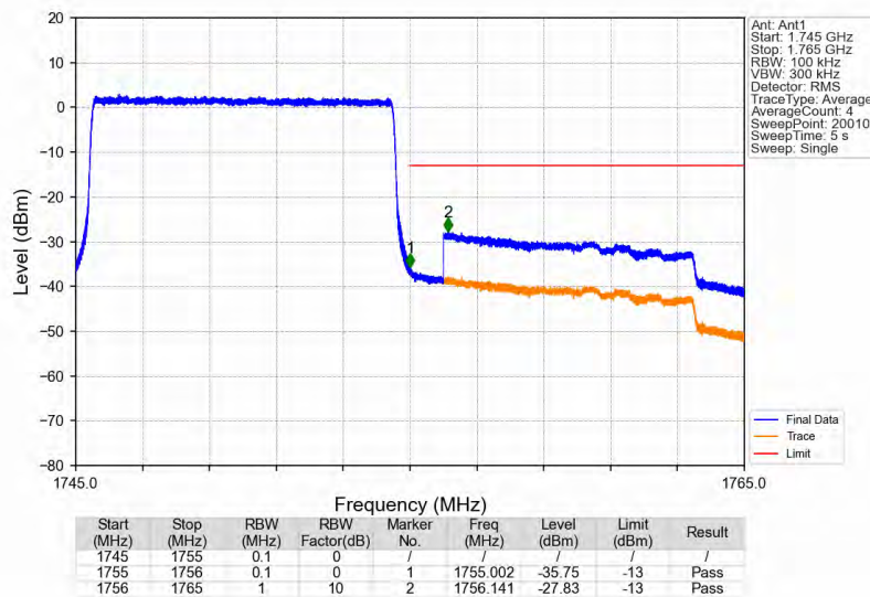
Band4_10MHz_QPSK_HCH_1750MHz_RB_50_0_NTNV
