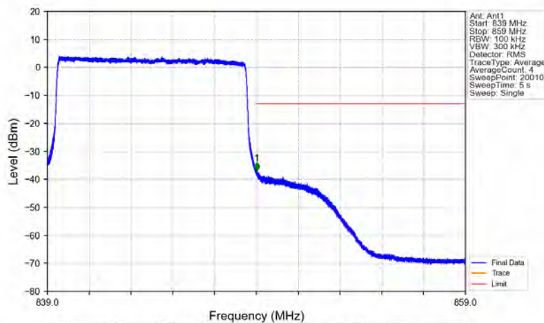
Band5_10MHz_QPSK_HCH_844MHz_RB_50_0_NTNV
