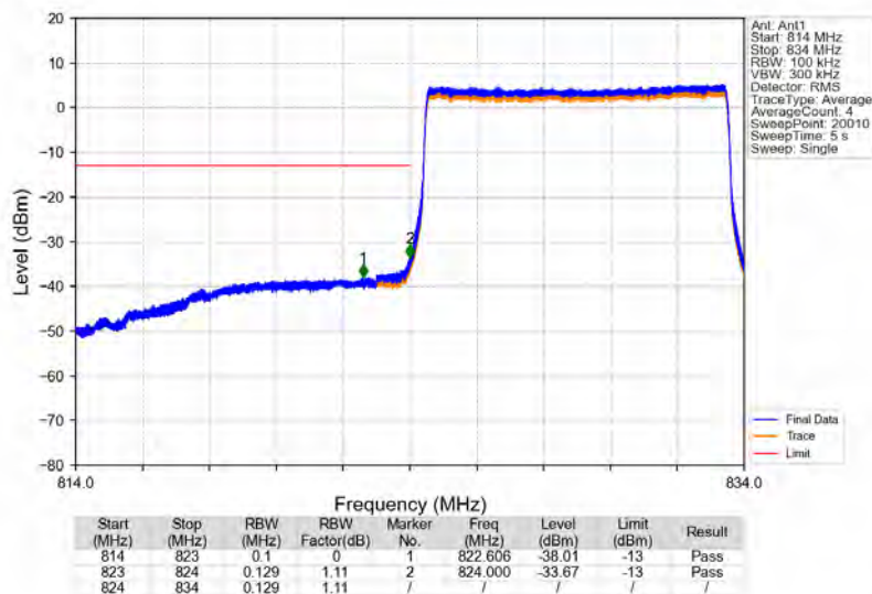
Band5_10MHz_QPSK_LCH_829MHz_RB_50_0_NTNV
