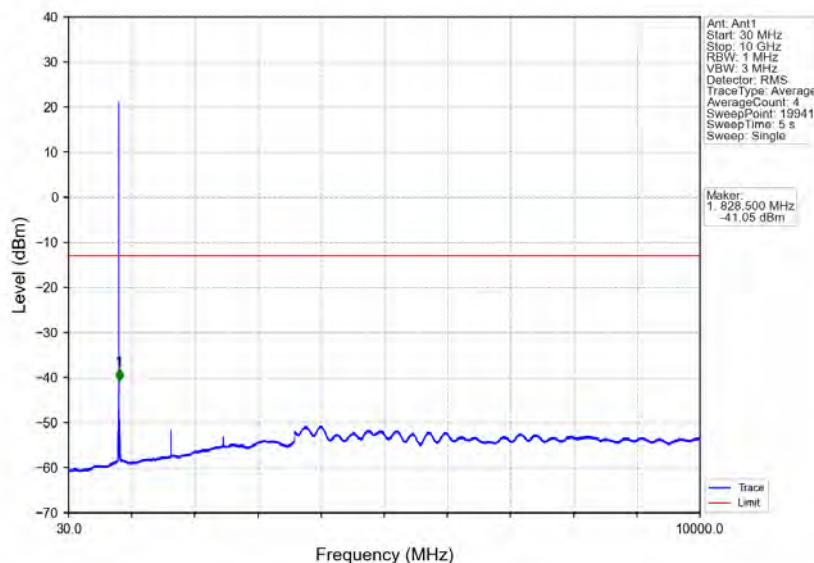
Band5 1.4MHz 16QAM LCH 824.7MHz RB 6 0 NTV
