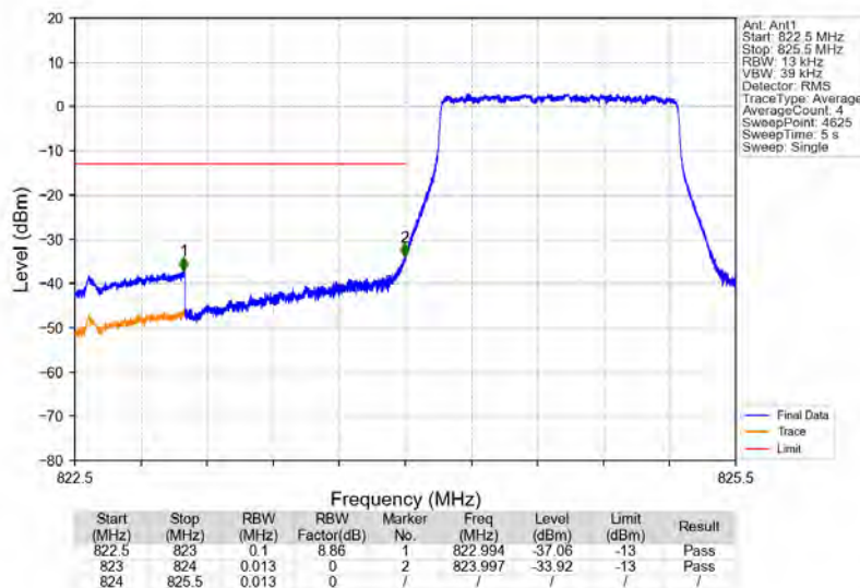
Band5 1.4MHz 16QAM LCH 824.7MHz RB 6 0 NTV
