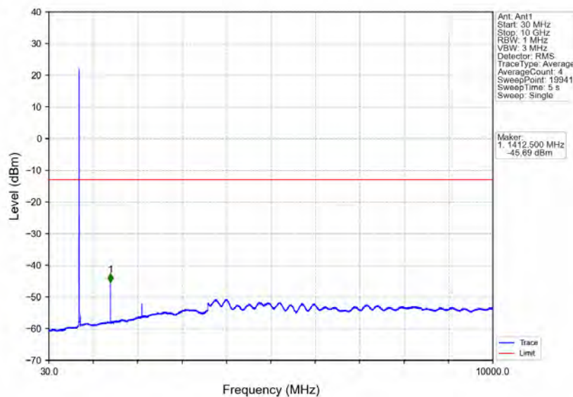
Band12_3MHz_QPSK_MCH_707.5MHz_RB_1_0_NTNV
