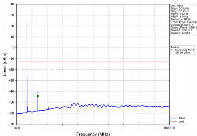
Band12_10MHz_QPSK_MCH_707.5MHz_RB_1_0_NTNV
