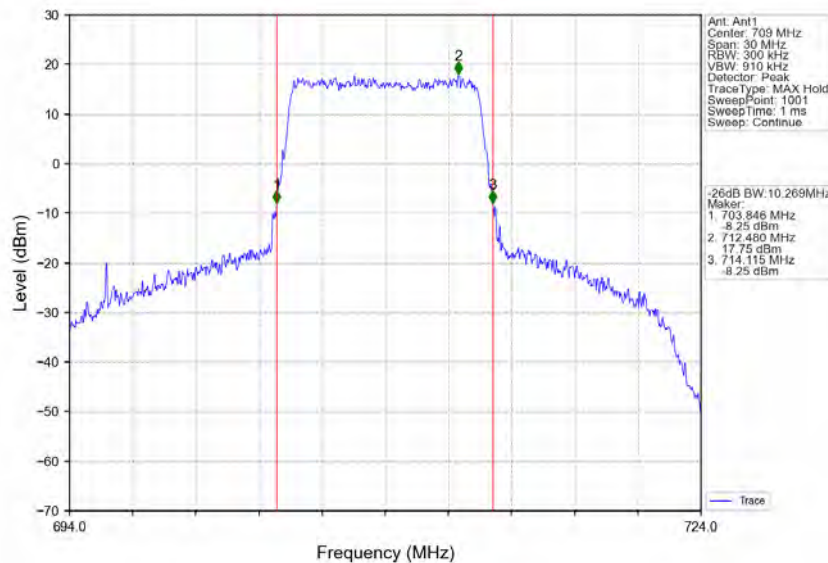
Band17_10MHz_QPSK_LCH_709MHz_RB_50_0_NTNV
