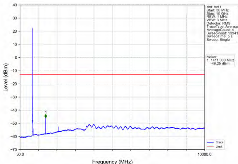
Band17_10MHz_QPSK_MCH_710MHz_RB_1_0_NTNV
