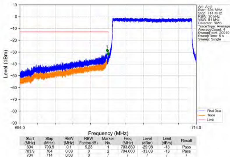
Band17_10MHz_QPSK_LCH_709MHz_RB_50_0_NTNV
