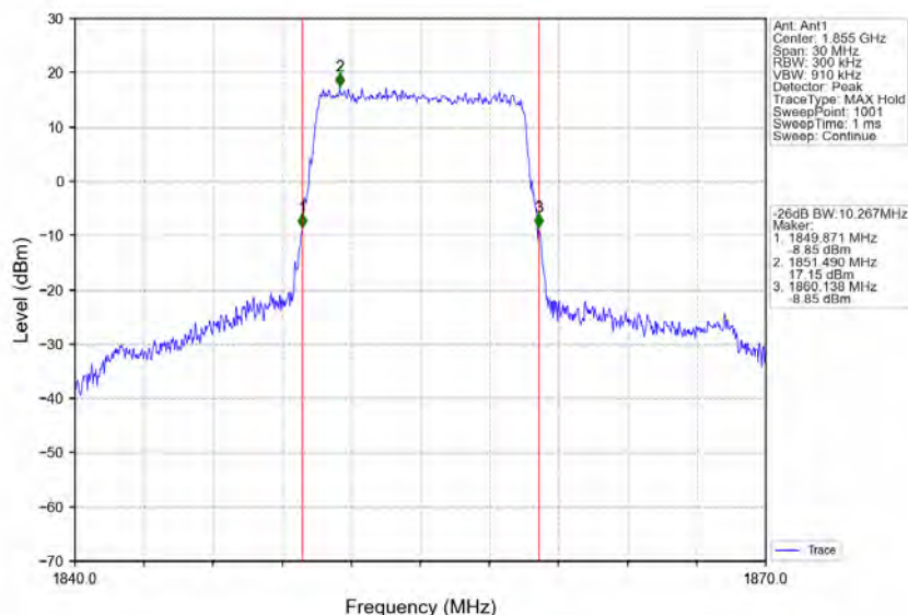
Band25_10MHz_QPSK_LCH_1855MHz_RB_50_0_NTNV
