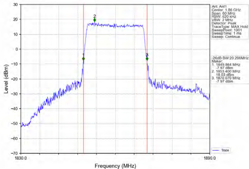
Band25_20MHz_QPSK_LCH_1860MHz_RB_100_0_NTNV
