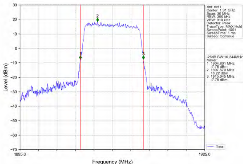
Band25_10MHz_QPSK_HCH_1910MHz_RB_50_0_NTNV
