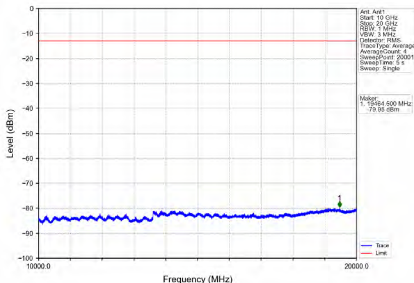
Band25_10MHz_QPSK_HCH_1910MHz_RB_1_0_NTNV
