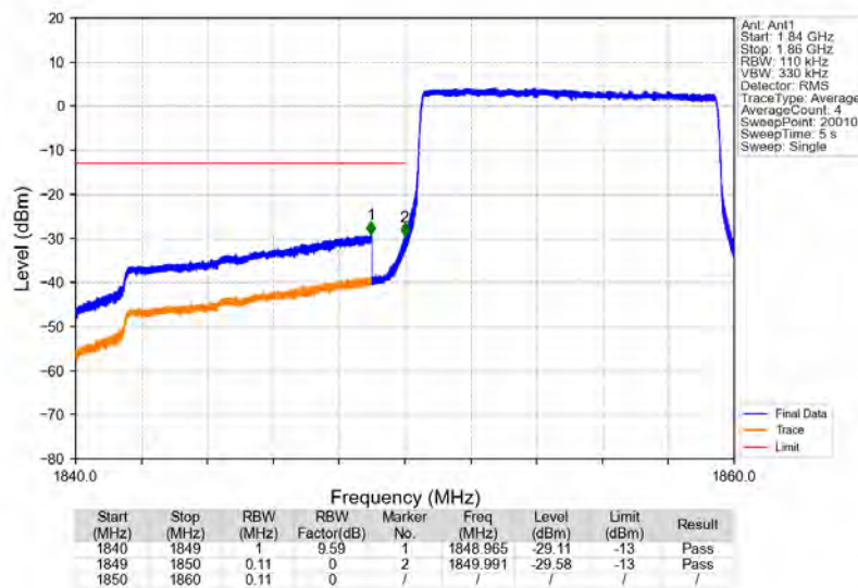
Band25_10MHz_QPSK_LCH_1855MHz_RB_50_0_NTNV
