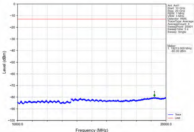
Band25_20MHz_QPSK_HCH_1905MHz_RB_1_0_NTNV
