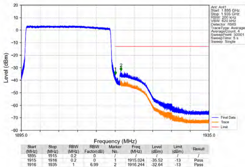
Band25_20MHz_QPSK_HCH_1905MHz_RB_100_0_NTNV
