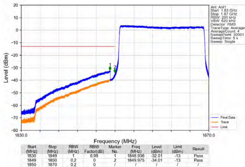
Band25_20MHz_QPSK_LCH_1860MHz_RB_100_0_NTNV
