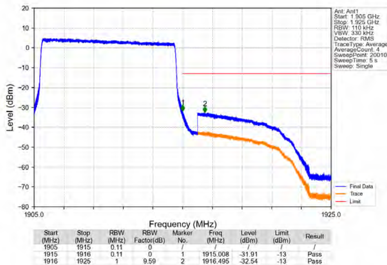
Band25_10MHz_QPSK_HCH_1910MHz_RB_50_0_NTNV
