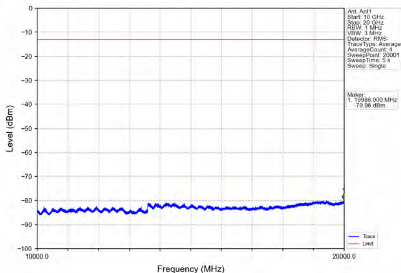
Band25_20MHz_QPSK_LCH_1860MHz_RB_100_0_NTNV
