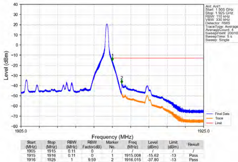
Band25_10MHz_QPSK_HCH_1910MHz_RB_1_49_NTNV
