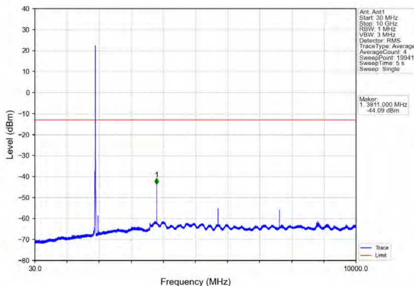
Band25_10MHz_QPSK_HCH_1910MHz_RB_1_0_NTNV
