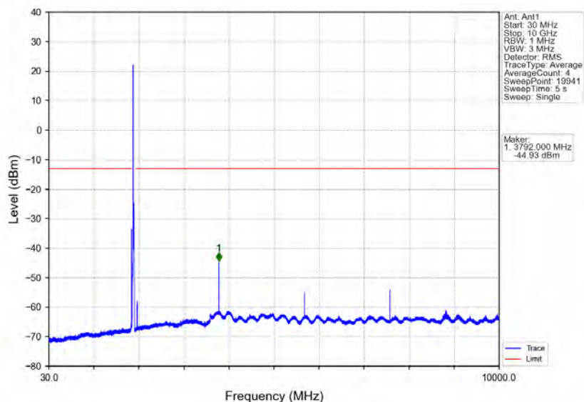
Band25_20MHz_QPSK_HCH_1905MHz_RB_1_0_NTNV
