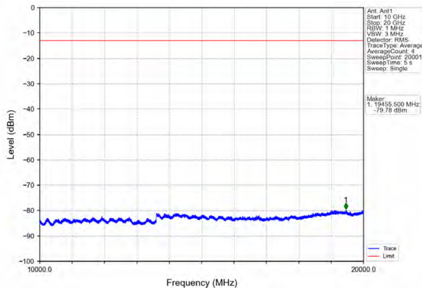
Band25_10MHz_QPSK_LCH_1855MHz_RB_50_0_NTNV
