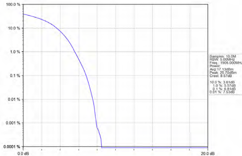
Band25_20MHz_QPSK_HCH_1905MHz_RB_100_0_NTNV
