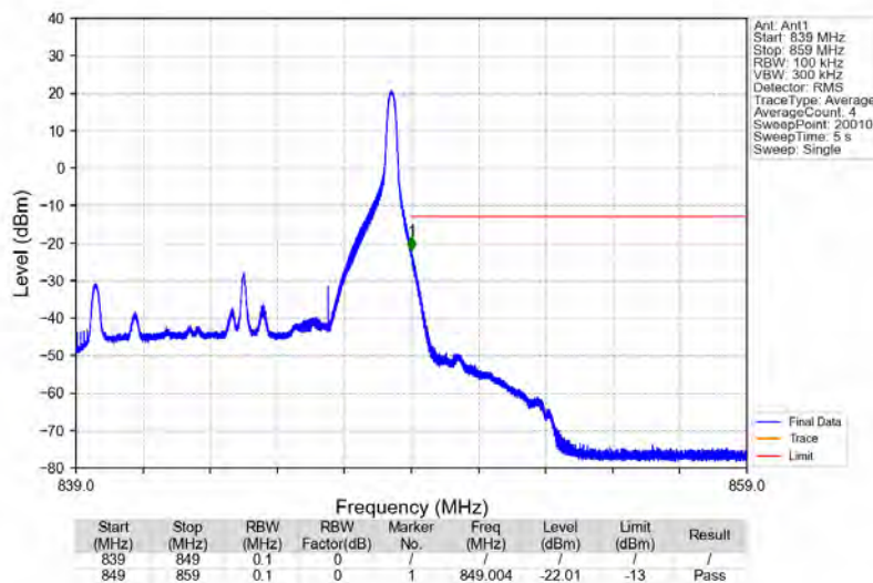
Band26b_10MHz_QPSK_HCH_844MHz_RB_1_49_NTNV
