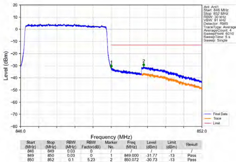
Band26b_3MHz_QPSK_HCH_847.5MHz_RB_15_0_NTNV
