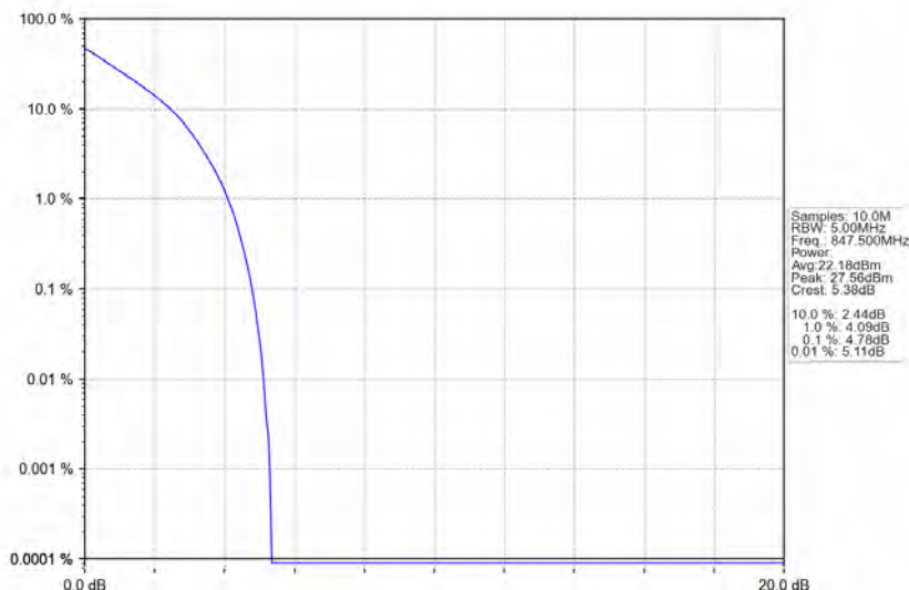
Band26b_3MHz_QPSK_HCH_847.5MHz_RB_15_0_NTNV
