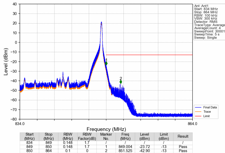
Band26c_15MHz_16QAM_HCH_841.5MHz_RB_1_74_NTNV
