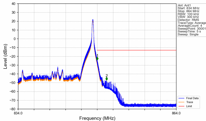
Band26c_15MHz_QPSK_HCH_841.5MHz_RB_1_74_NTNV
