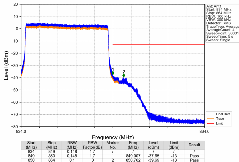
Band26c_15MHz_QPSK_HCH_841.5MHz_RB_75_0_NTNV
