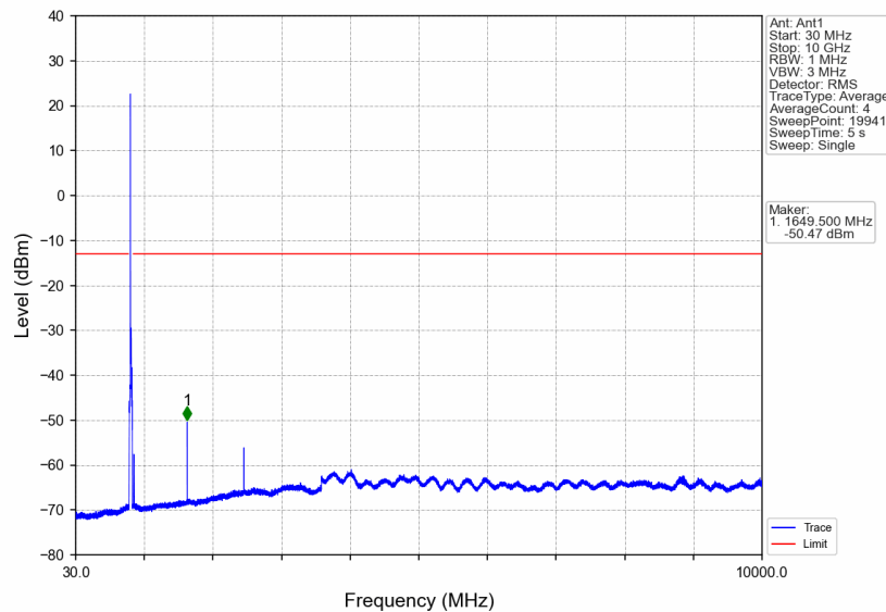
Band26c_15MHz_QPSK_MCH_831.5MHz_RB_1_0_NTNV
