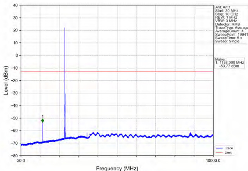
Band30_10MHz_QPSK_HCH_2310MHz_RB_1_0_NTNV
