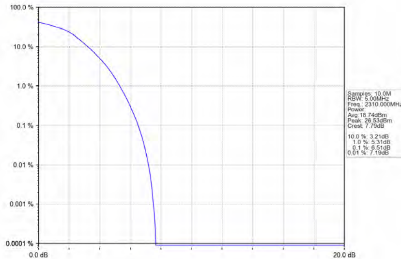
Band30_10MHz_16QAM_LCH_2310MHz_RB_50_0_NTNV
