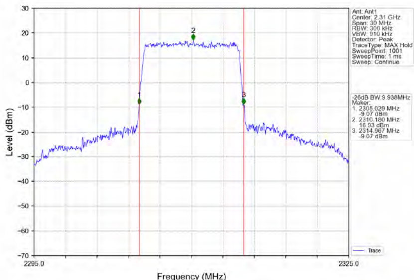
Band30_10MHz_QPSK_HCH_2310MHz_RB_50_0_NTNV
