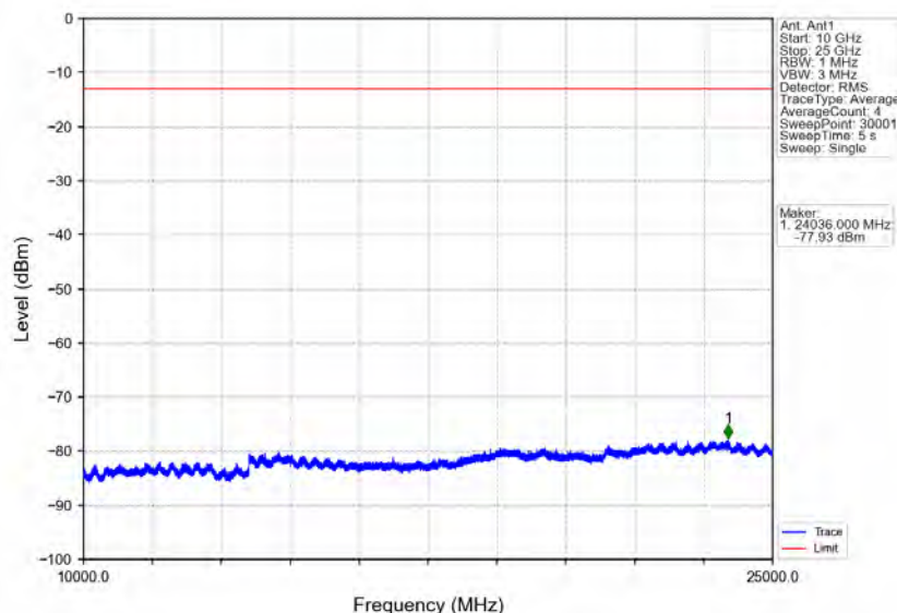
Band30_10MHz_QPSK_HCH_2310MHz_RB_1_0_NTNV
