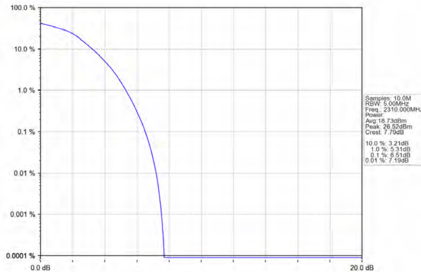
Band30_10MHz_16QAM_MCH_2310MHz_RB_50_0_NTNV
