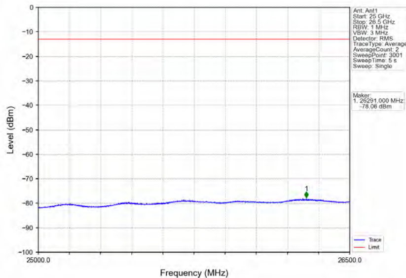
Band30_5MHz_QPSK_LCH_2307.5MHz_RB_1_0_NTNV
