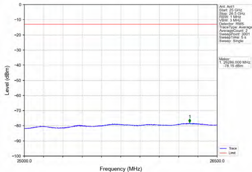
Band30_10MHz_QPSK_HCH_2310MHz_RB_1_49_NTNV
