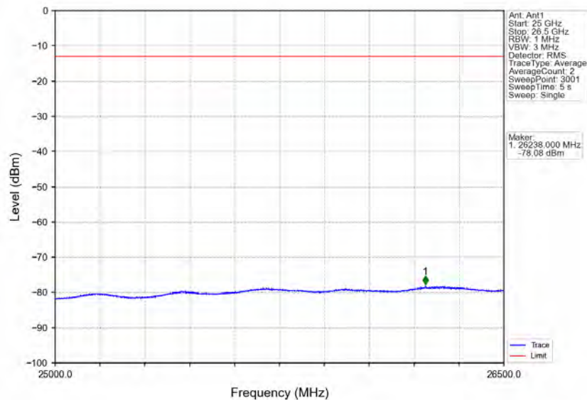
Band30_10MHz_QPSK_MCH_2310MHz_RB_1_0_NTNV
