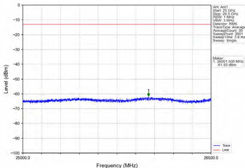
Band30_10MHz_16QAM_LCH_2310MHz_RB_50_0_NTNV
