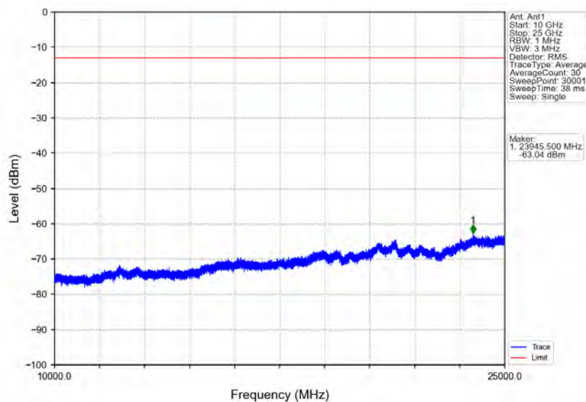
Band30_10MHz_16QAM_LCH_2310MHz_RB_1_0_NTNV
