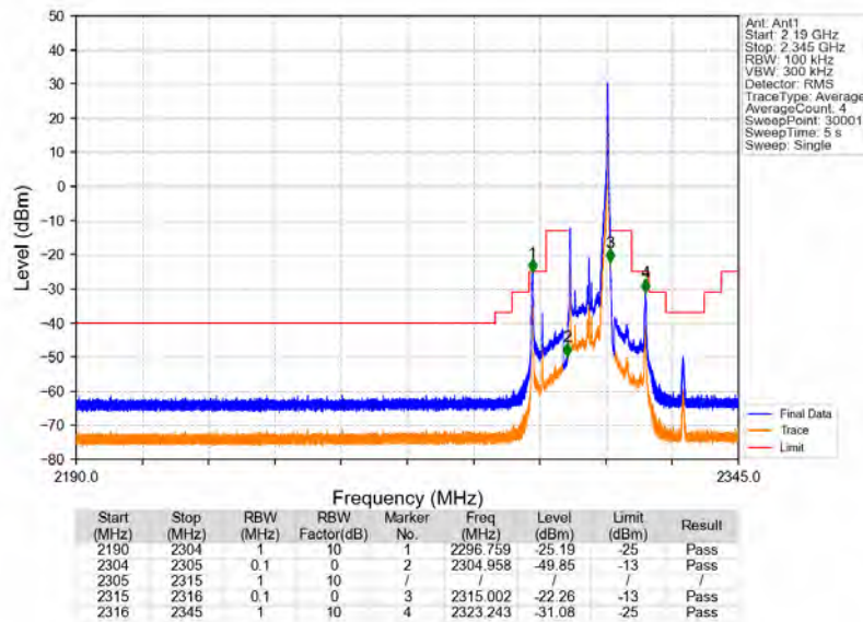
Band30_10MHz_QPSK_HCH_2310MHz_RB_1_49_NTNV
