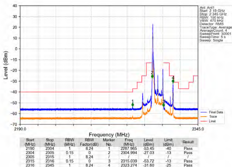
Band30_10MHz_16QAM_LCH_2310MHz_RB_1_0_NTNV
