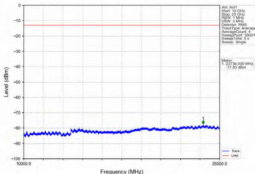
Band30_10MHz_16QAM_MCH_2310MHz_RB_1_0_NTNV
