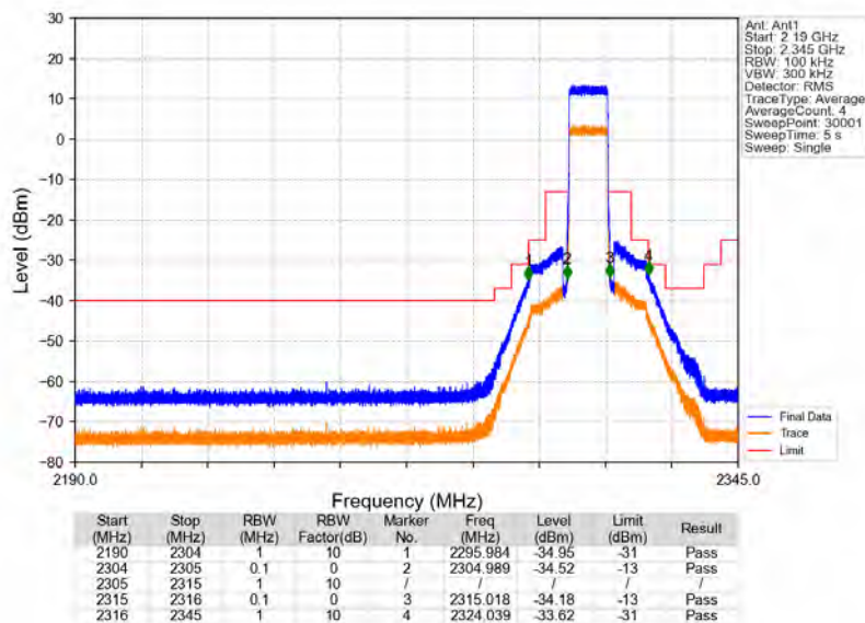
Band30_10MHz_16QAM_LCH_2310MHz_RB_1_0_NTNV
