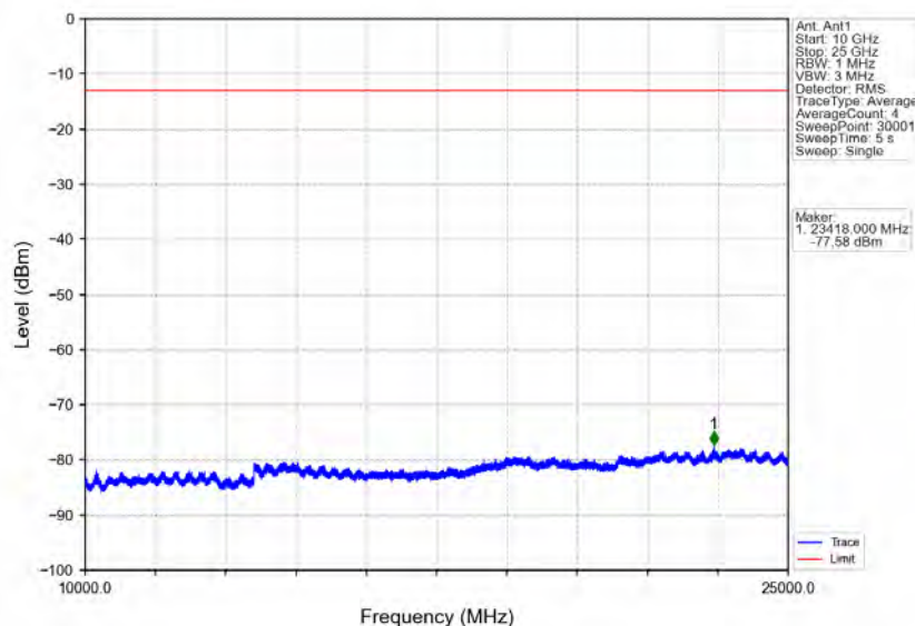
Band30_5MHz_QPSK_MCH_2310MHz_RB_1_0_NTNV
