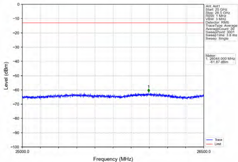
Band30_10MHz_QPSK_LCH_2310MHz_RB_1_0_NTNV
