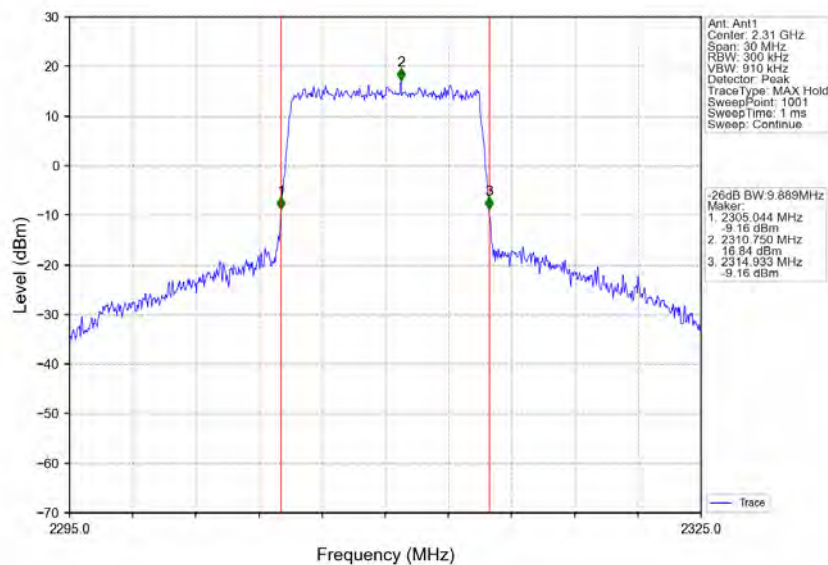
Band30_10MHz_16QAM_MCH_2310MHz_RB_50_0_NTNV
