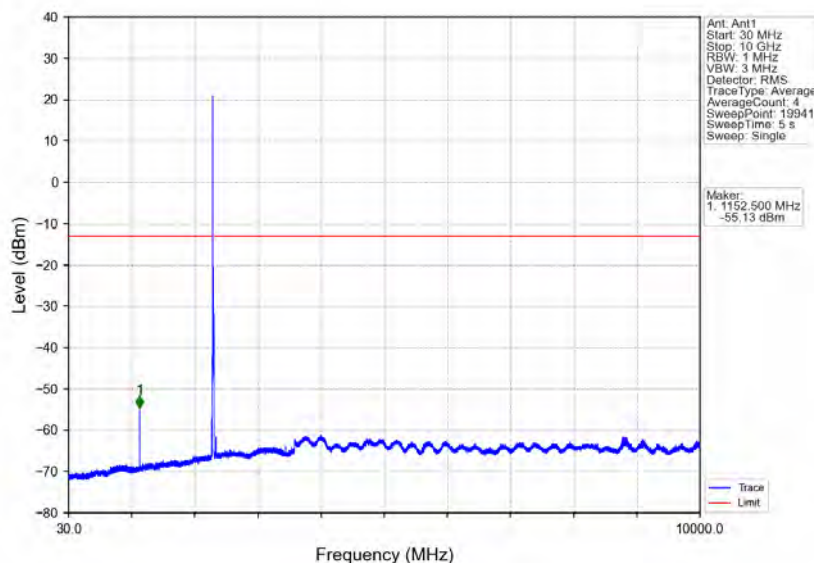
Band30_10MHz_16QAM_MCH_2310MHz_RB_1_0_NTNV
