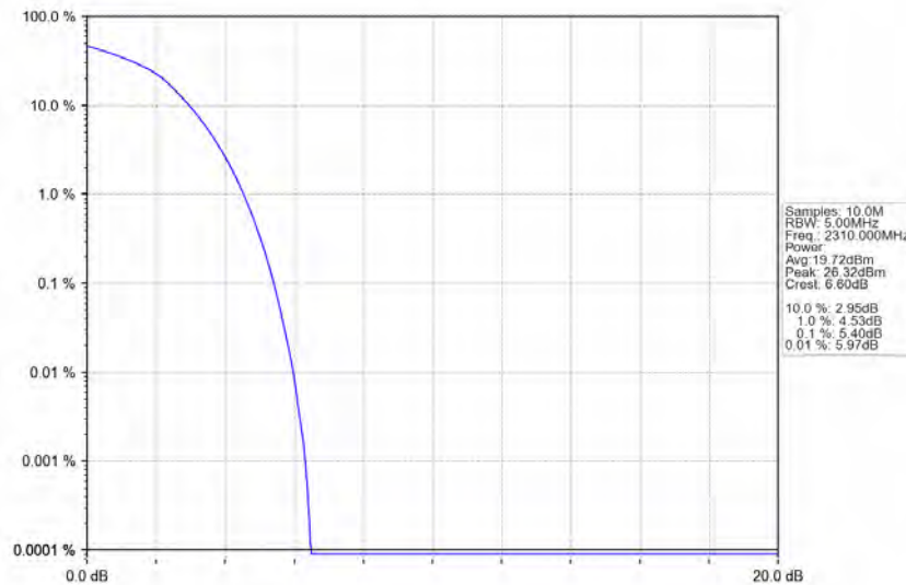
Band30_10MHz_QPSK_HCH_2310MHz_RB_50_0_NTNV
