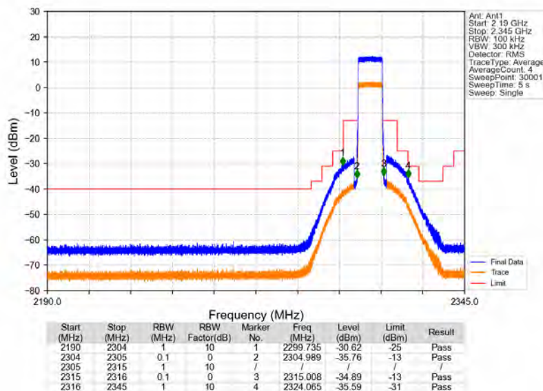
Band30_10MHz_16QAM_LCH_2310MHz_RB_50_0_NTNV
