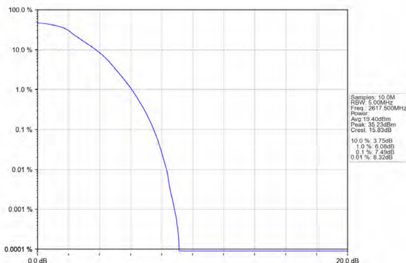
Band38 5MHz QPSK HCH 2617.5MHz RB 25 0 NTNV
