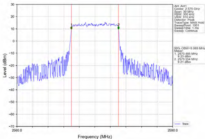
Band38 10MHz 64QAM LCH 2575MHz RB 50 0 NTNV
