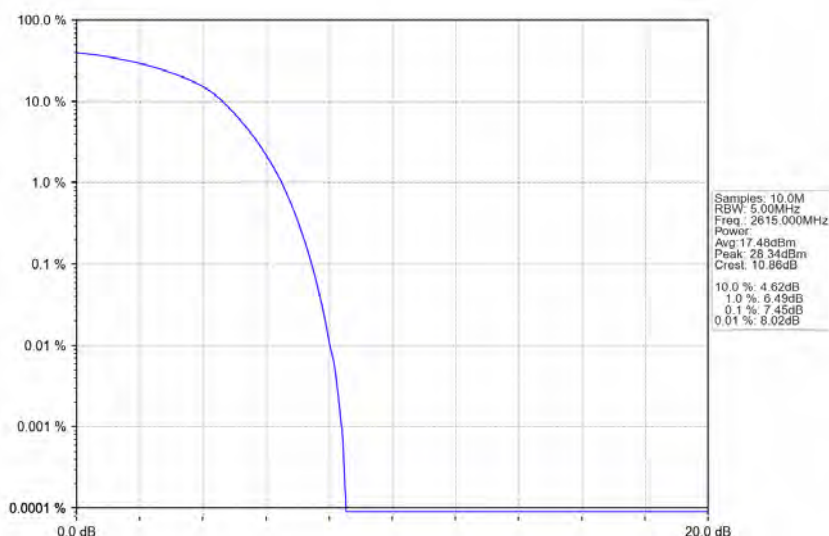
Band38 10MHz QPSK HCH 2615MHz RB 50 0 NTV
