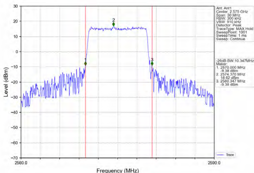
Band38_10MHz_QPSK_LCH 2575MHz_RB_50_0 NTN
