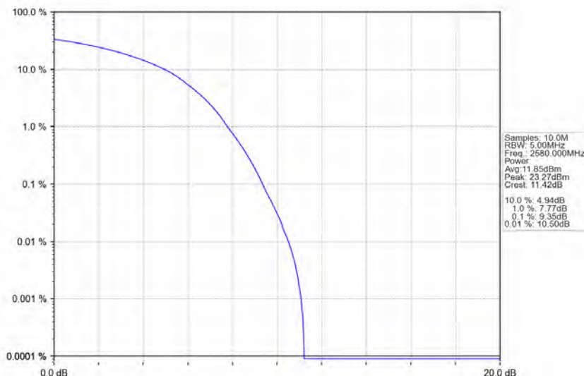
Band38 20MHz 64QAM LCH 2580MHz RB 100 0 NTNV
