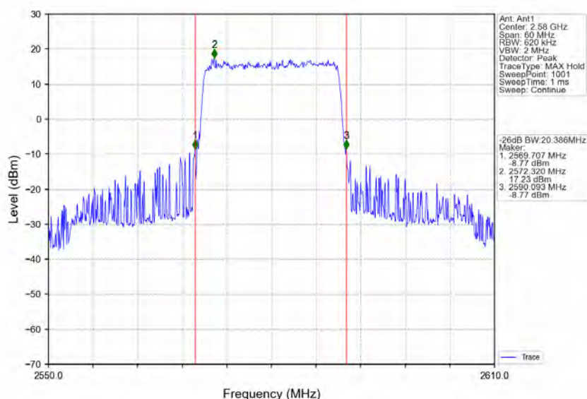
Band38 20MHz QPSK LCH 2580MHz RB 100 0 NTNV
