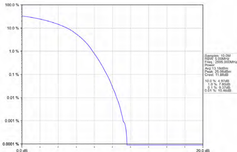
Band38_20MHz_16QAM_MCH_2595MHz_RB_100_0_NTNV
