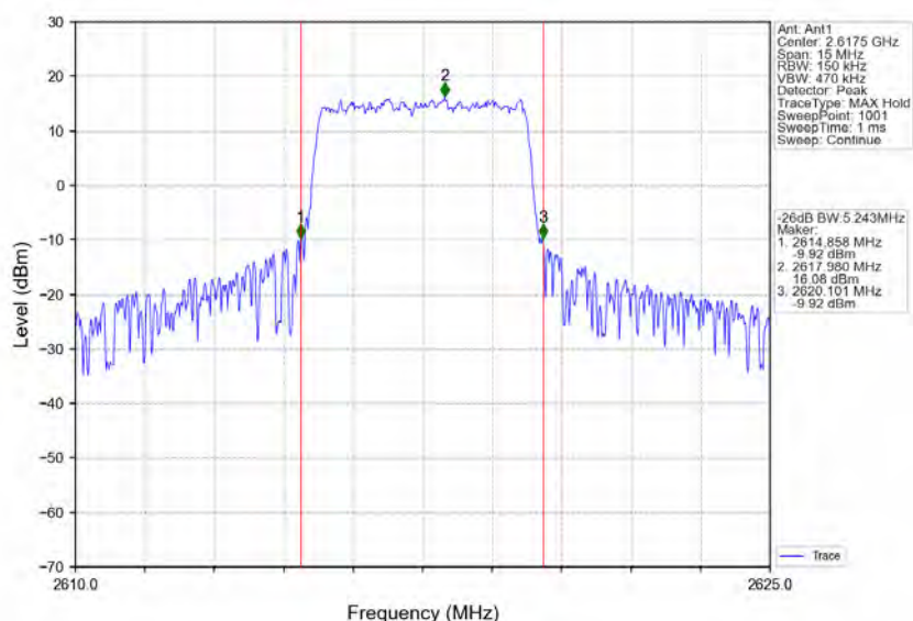
Band38 5MHz 16QAM HCH 2617.5MHz RB 25 0 NTNV
