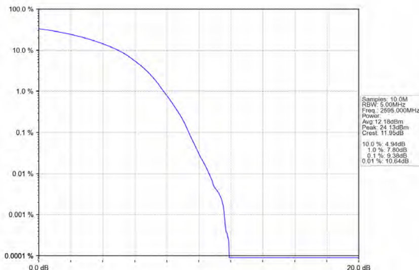
Band38_20MHz 64QAM MCH 2595MHz RB 100 0 NTNV
