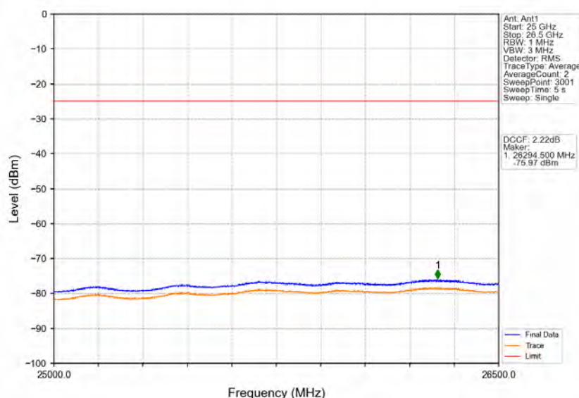
Band38_20MHz_16QAM_HCH_2610MHz_RB_1_0_NTNV
