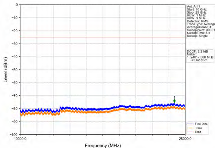
Band38_20MHz_16QAM_LCH_2580MHz_RB_1_0_NTV
