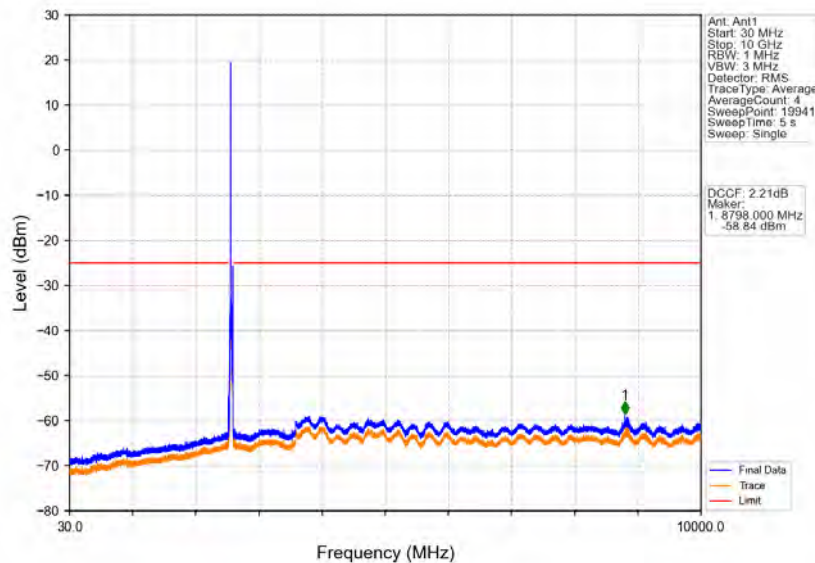
Band38_20MHz_16QAM_LCH_2580MHz_RB_1_0_NTV
