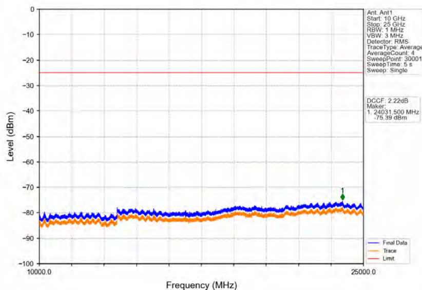
Band38_20MHz_16QAM_MCH_2595MHz_RB_1_0_NTNV
