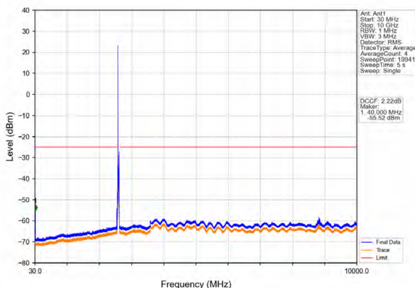
Band38_20MHz_16QAM_HCH_2610MHz_RB_1_0_NTNV
