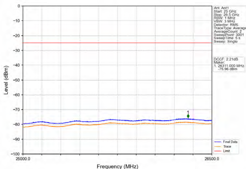
Band38_10MHz_QPSK_HCH_2615MHz_RB_1_49_NTNV
