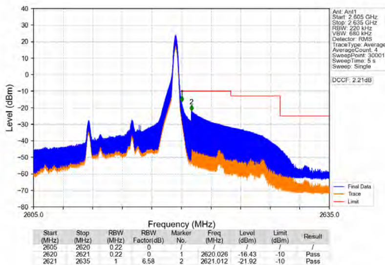
Band38_10MHz_QPSK_HCH_2615MHz_RB_1_49_NTNV
