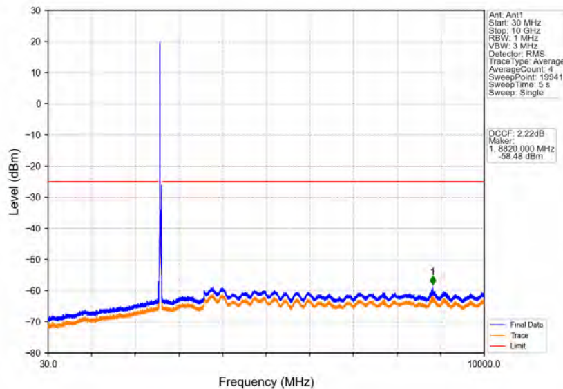
Band38_20MHz_16QAM_MCH_2595MHz_RB_1_0_NTNV
