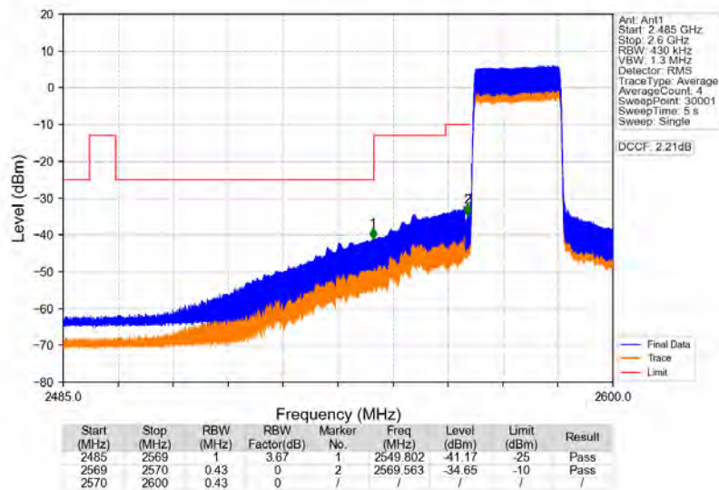
Band38_20MHz_64QAM_LCH_2580MHz_RB_100_0_NTNV
