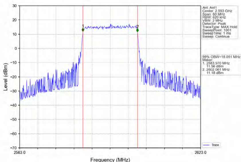
Band41_20MHz_16QAM_MCH_2593MHz_RB_100_0_NTNV
