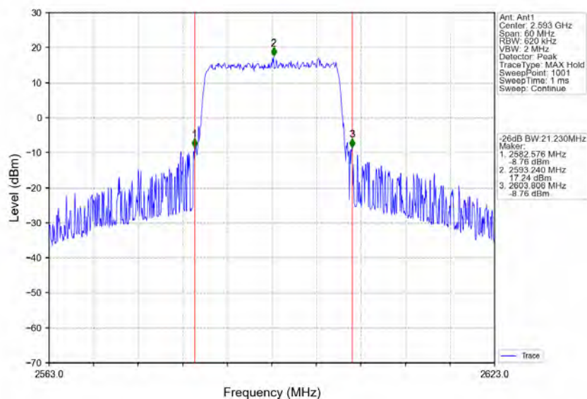
Band41 20MHz 16QAM MCH 2593MHz RB 100 0 NTNV
