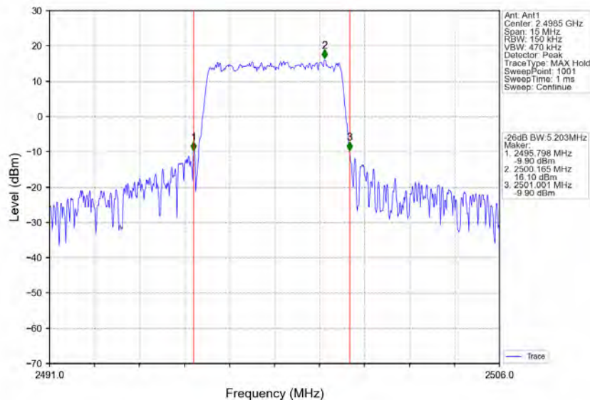
Band41 5MHz 16QAM LCH 2498.5MHz RB 25 0 NTV
