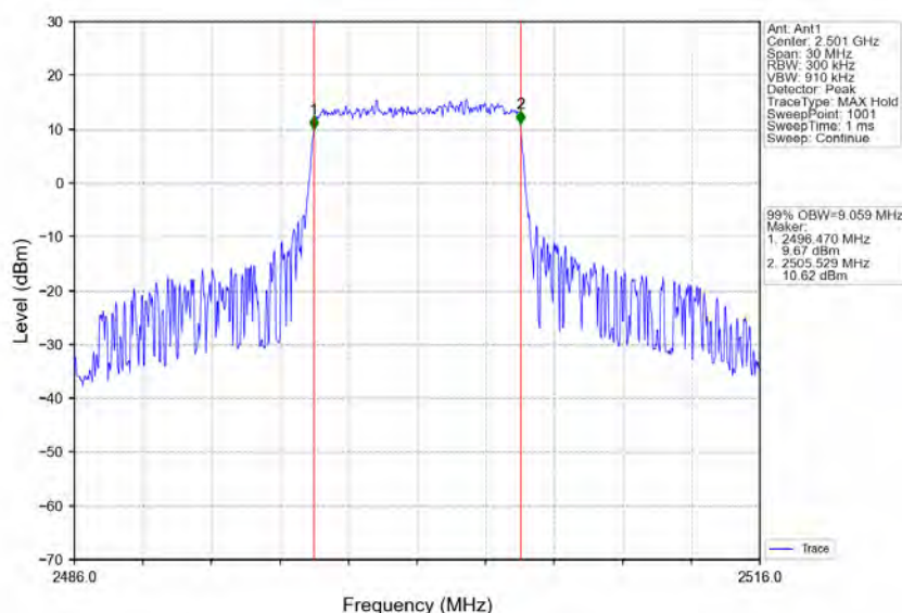
Band41 10MHz 64QAM LCH 2501MHz RB 50 0 NTNV
