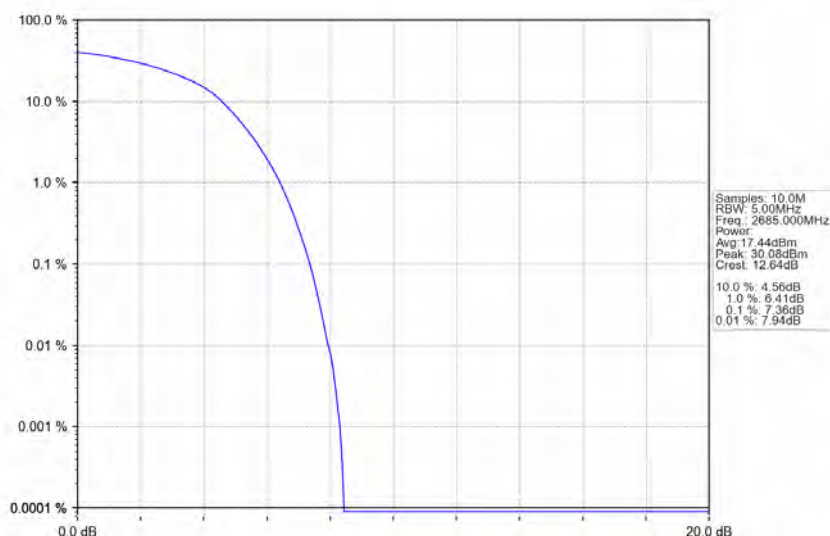
Band41_10MHz_QPSK_HCH_2685MHz_RB_50_0_NTNV
