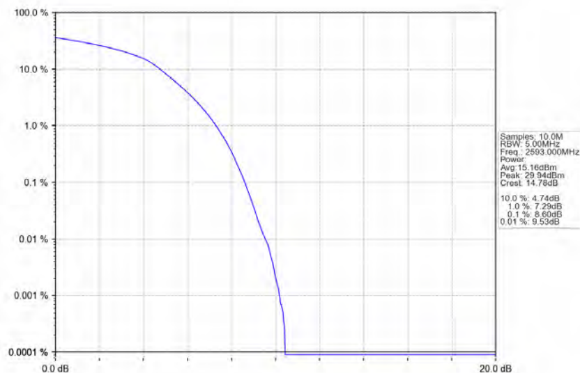
Band41 10MHz 64QAM MCH 2593MHz RB 50 0 NTN
