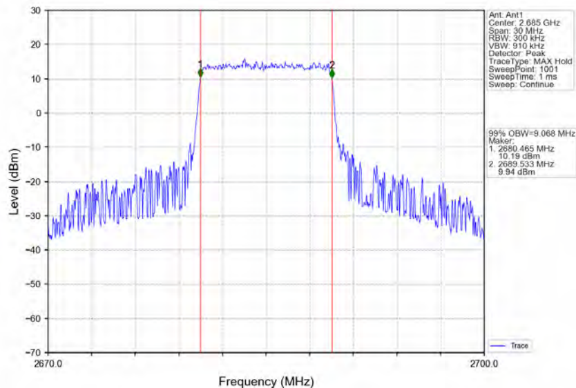
Band41 10MHz 64QAM HCH 2685MHz RB 50 0 NTNV
