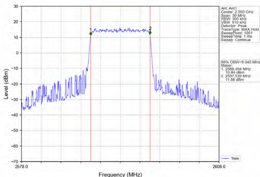
Band41 10MHz 16QAM MCH 2593MHz RB 50 0 NTNV
