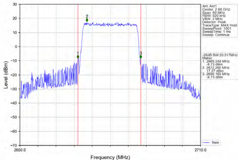
Band41 20MHz QPSK HCH 2680MHz RB 100 0 NTNV
