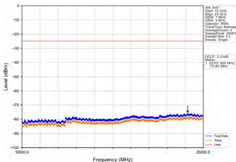
Band41_15MHz_QPSK_MCH_2593MHz_RB_1_0_NTNV
