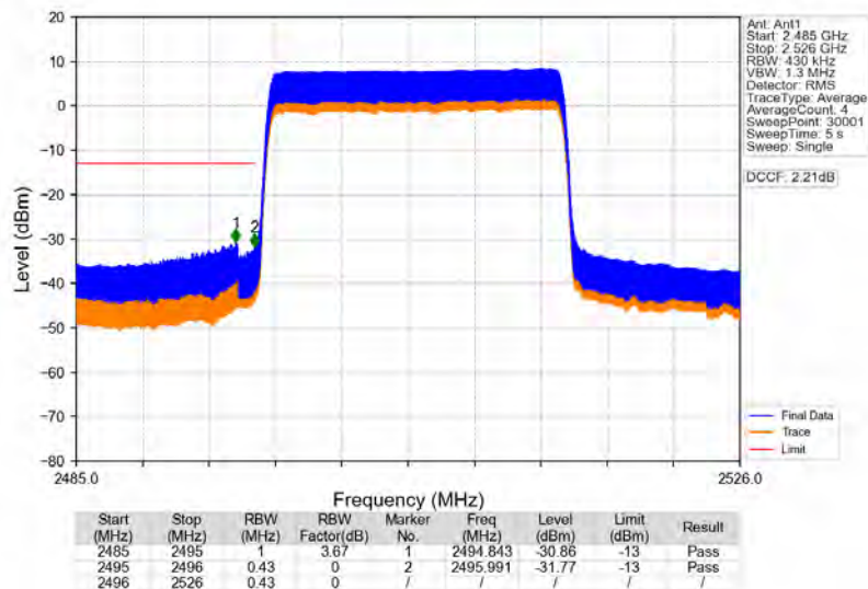
Band41_20MHz_QPSK_LCH_2506MHz_RB_100_0_NTNV
