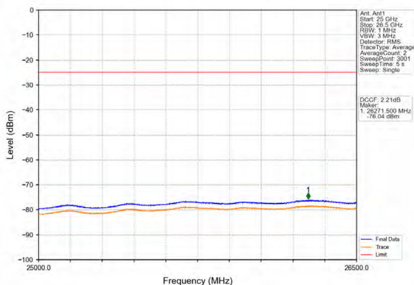
Band41 5MHz QPSK HCH 2687.5MHz RB 1 24 NTNV
