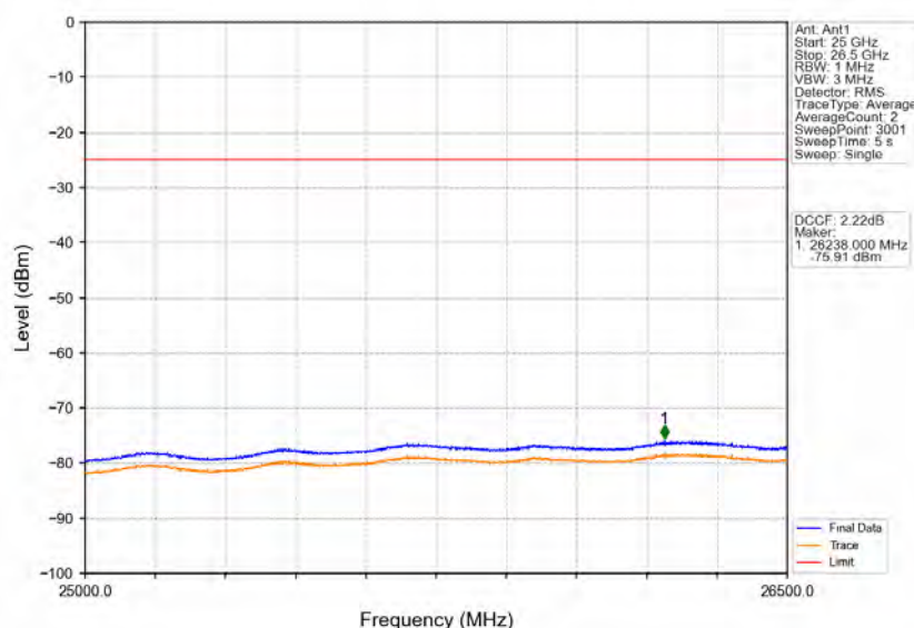
Band41 20MHz QPSK MCH 2593MHz RB 1 0 NTNV
