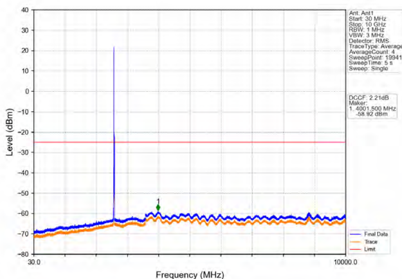
Band41_10MHz_16QAM_MCH_2593MHz_RB_1_0_NTNV
