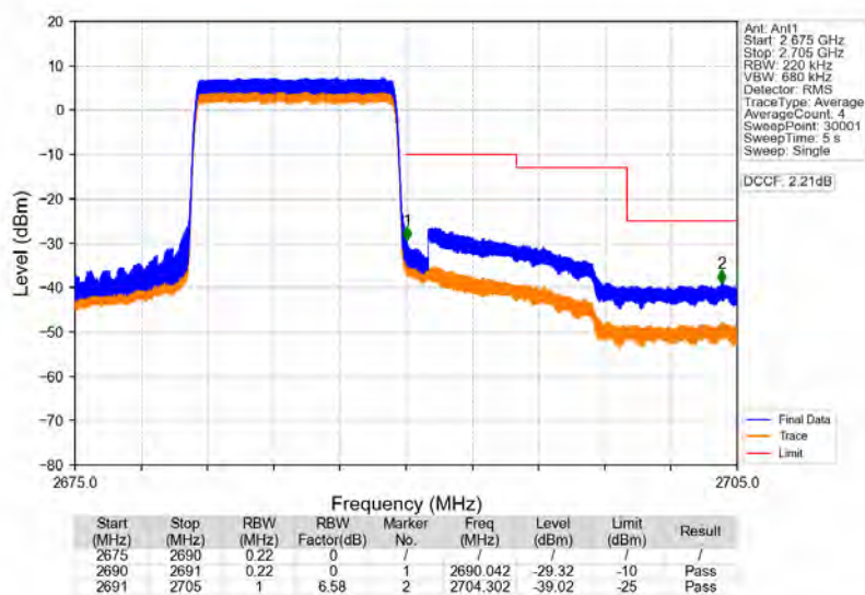
Band41 10MHz QPSK HCH 2685MHz RB 50 0 NTNV
