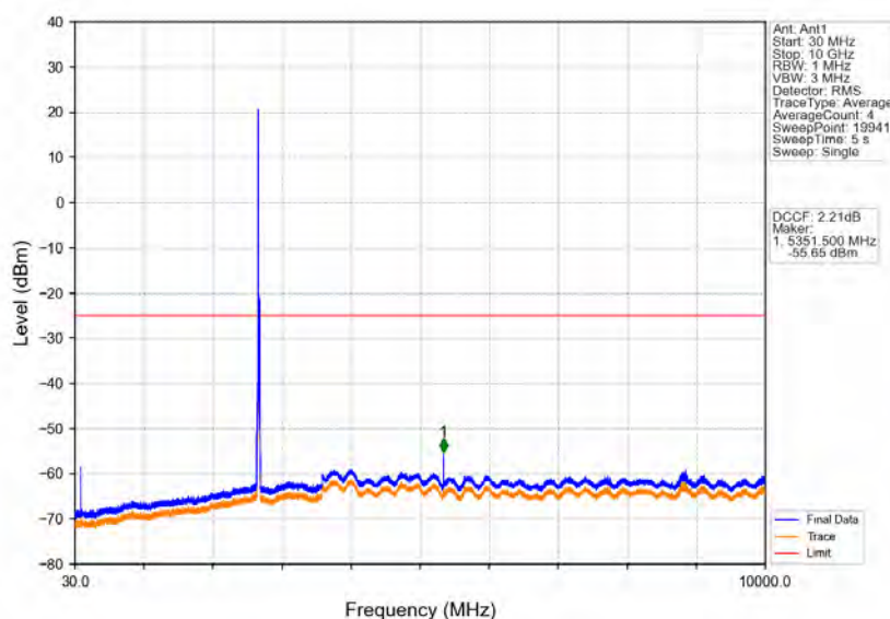
Band41_15MHz_QPSK_HCH_2682.5MHz_RB_1_0_NTNV
