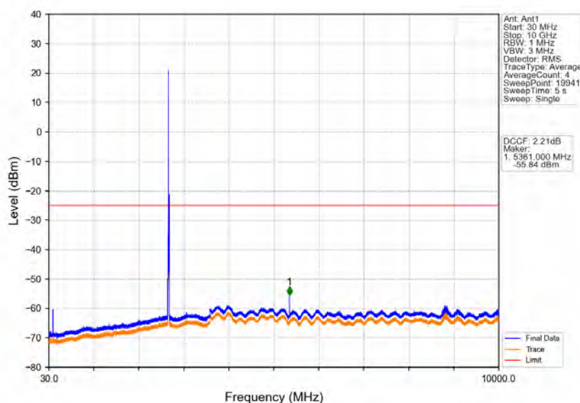
Band41_10MHz_QPSK_HCH_2685MHz_RB_1_0_NTNV
