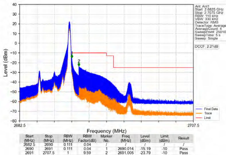
Band41 5MHz QPSK HCH 2687.5MHz RB 1 24 NTNV
