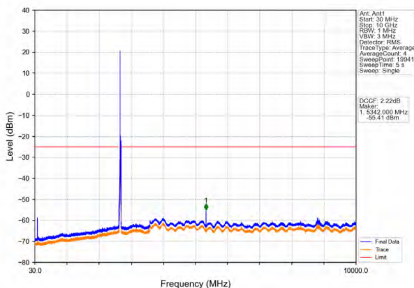
Band41 20MHz QPSK HCH 2680MHz RB 1 0 NTNV
