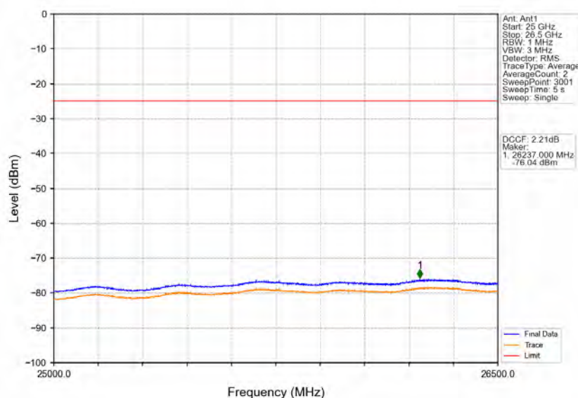
Band41 10MHz 64QAM HCH 2685MHz RB 1 49 NTNV
