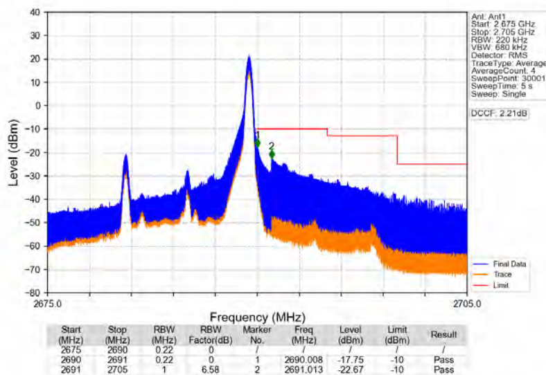
Band41 10MHz 64QAM HCH 2685MHz RB 1 49 NTNV
