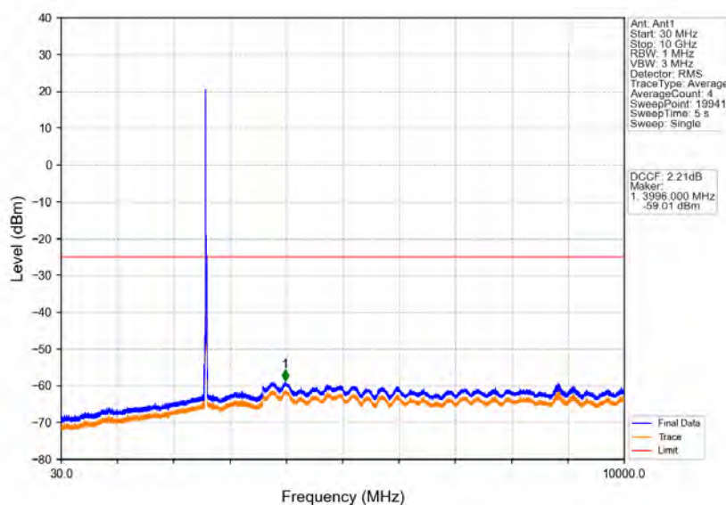
Band41_15MHz_QPSK_MCH_2593MHz_RB_1_0_NTNV
