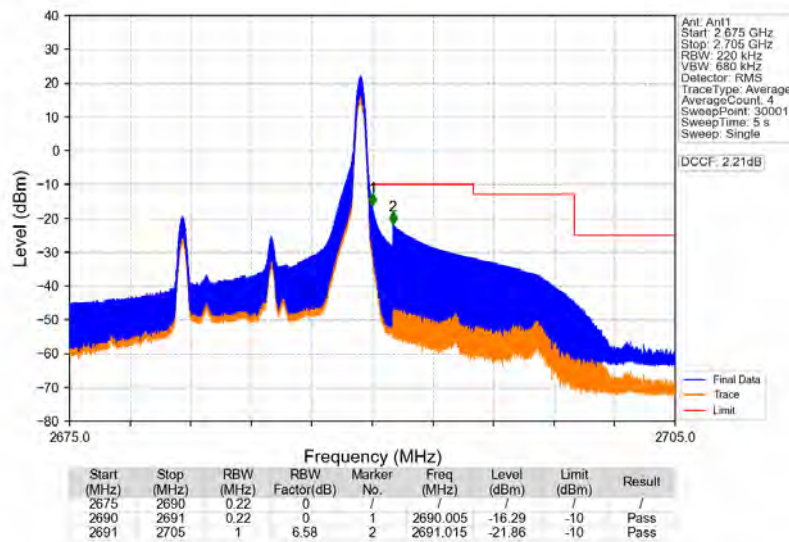
Band41 10MHz 16QAM HCH 2685MHz RB 1 49 NTNV
