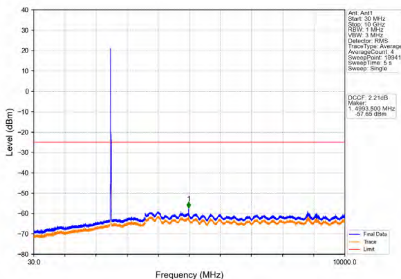
Band41_10MHz_16QAM_LCH_2501MHz_RB_1_0_NTNV
