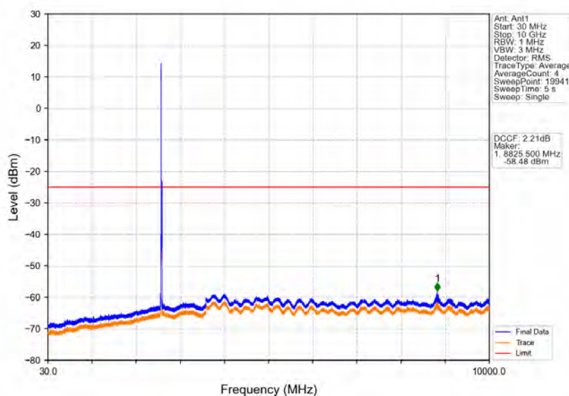
Band41_10MHz_QPSK_MCH_2593MHz_RB_1_0_NTNV
