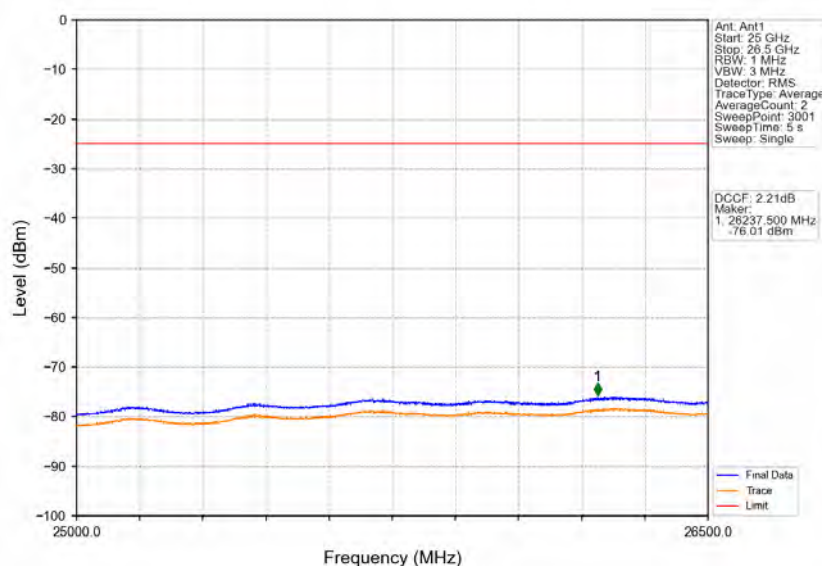
Band41_10MHz_16QAM_LCH_2501MHz_RB_50_0_NTNV
