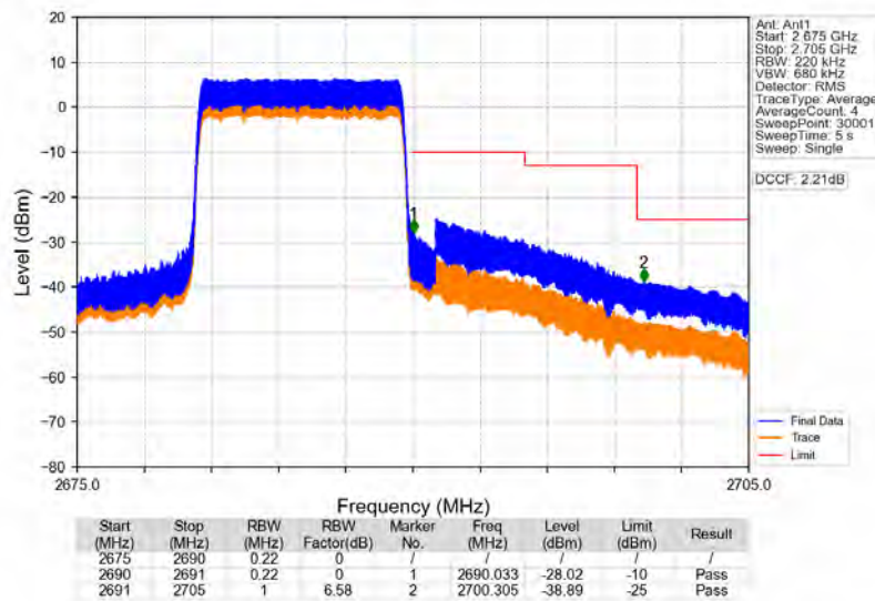
Band41 10MHz 16QAM HCH 2685MHz RB 50 0 NTNV
