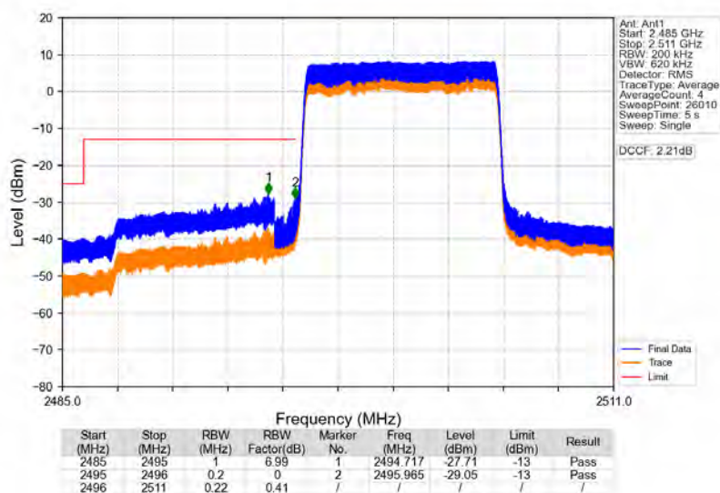
Band41_10MHz_QPSK_LCH_2501MHz_RB_50_0_NTNV
