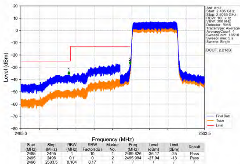
Band41 5MHz QPSK LCH 2498.5MHz RB 25 0 NTN
