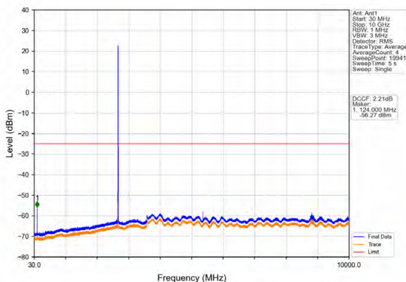
Band41_5MHz_QPSK_HCH_2687.5MHz_RB_1_0_NTNV
