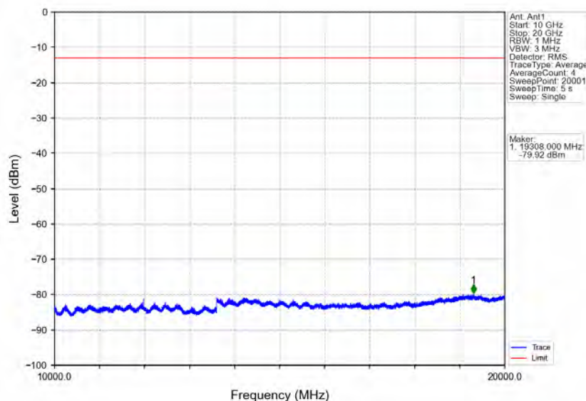
Band66_20MHz_QPSK_LCH_1720MHz_RB_100_0_NTNV
