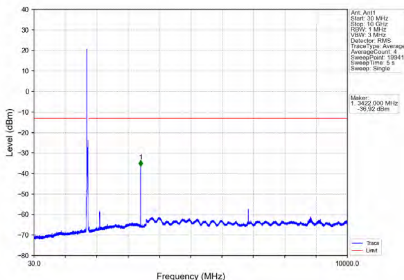
Band66_20MHz_16QAM_LCH_1720MHz_RB_1_0_NTNV
