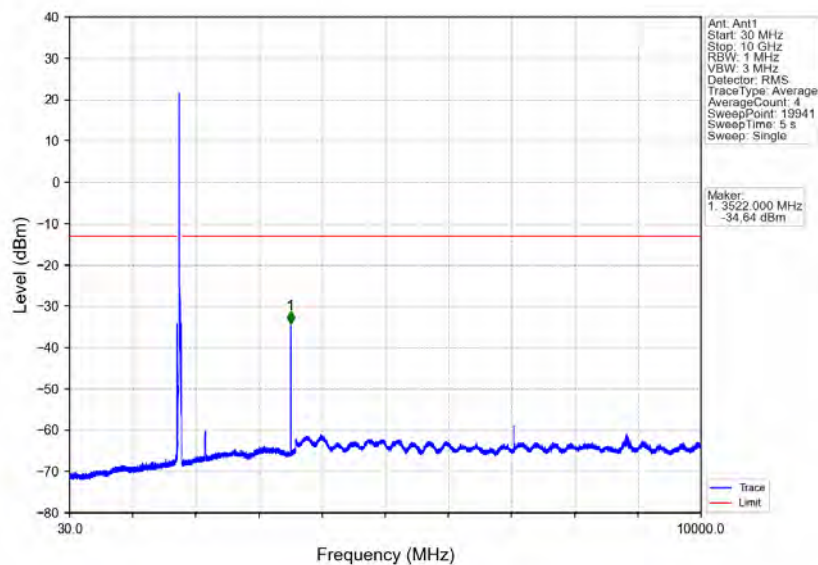
Band66_20MHz_QPSK_HCH_1770MHz_RB_1_0_NTNV
