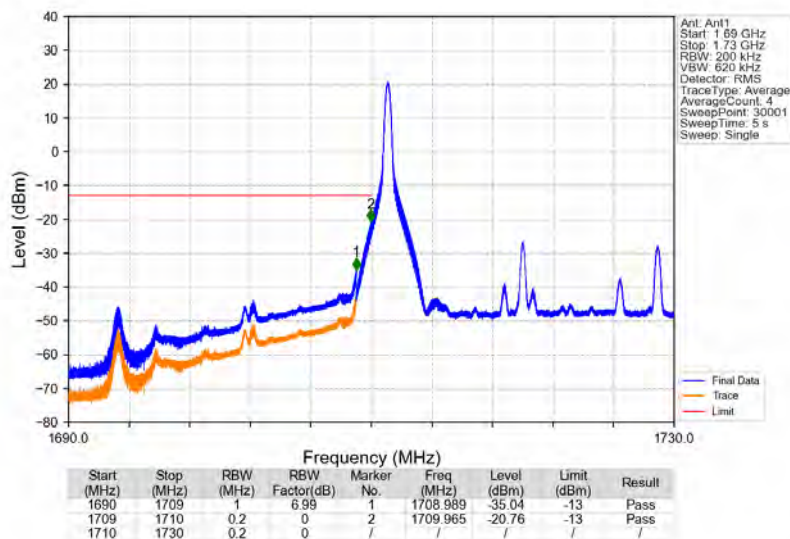
Band66_20MHz_16QAM_LCH_1720MHz_RB_1_0_NTNV
