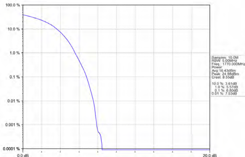
Band66_20MHz_QPSK_HCH_1770MHz_RB_100_0_NTNV
