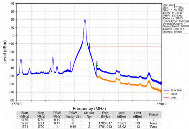
Band66_10MHz_QPSK_HCH_1775MHz_RB_1_49_NTNV
