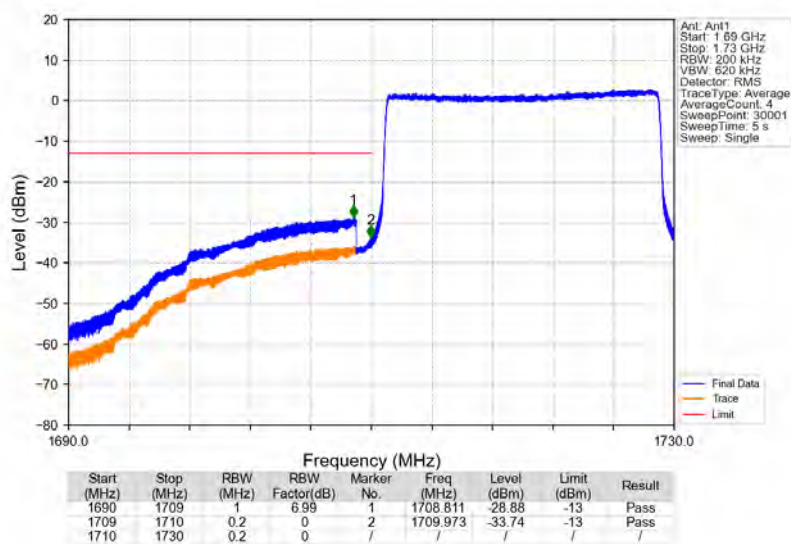
Band66_20MHz_16QAM_LCH_1720MHz_RB_100_0_NTNV
