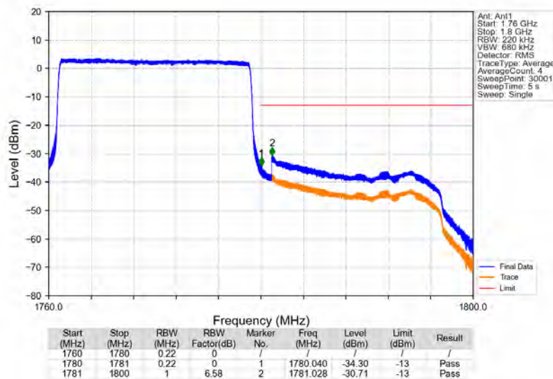
Band66_20MHz_QPSK_HCH_1770MHz_RB_100_0_NTNV
