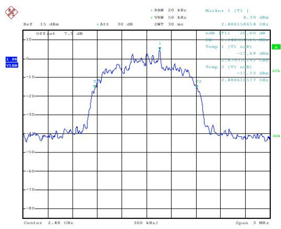
20dB Bandwidth: \pi/4 DQPSK, Ch78
