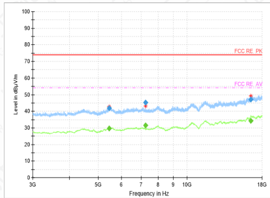
RSE-11G-CH1-3GHz-18GHz
