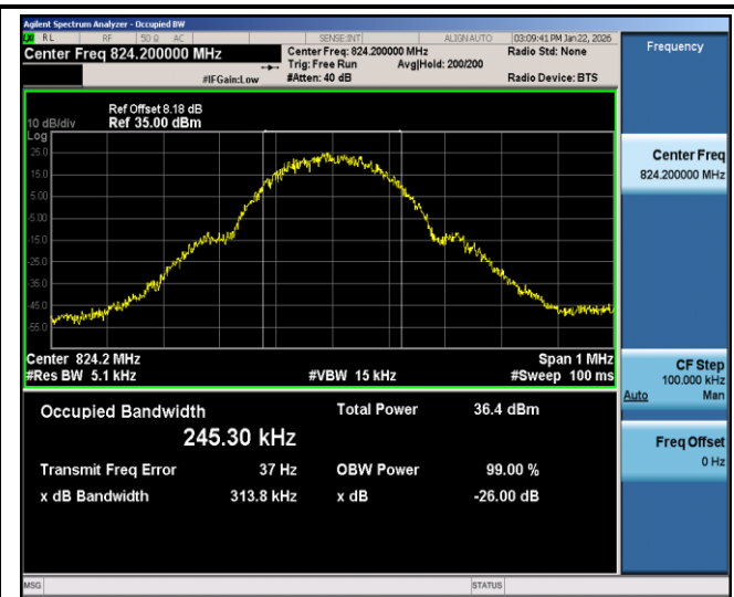
GPRS850-128-3-0.3138
