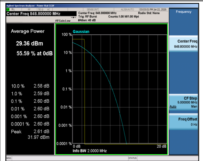
GPRS850-251-3
