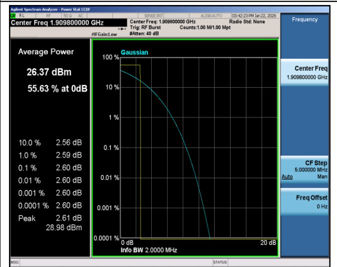
GSM1900-810-0
