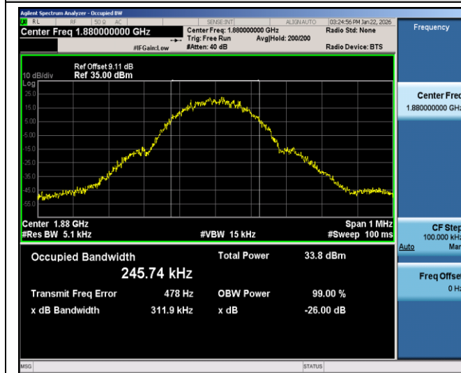
GSM1900-661-0-0.3119
