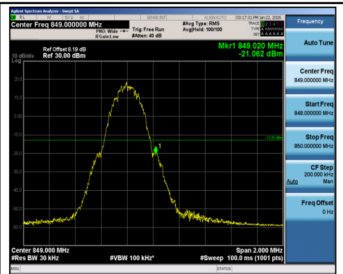
GPRS850-251-3
