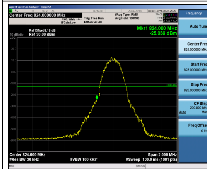
EGPRS850-128-8
