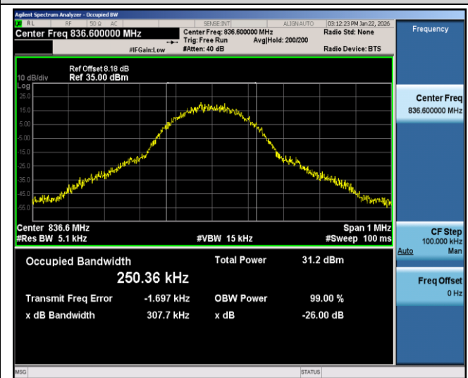
EGPRS850-190-8-0.3077
