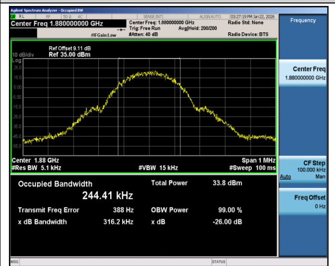
GPRS1900-661-0-0.3162
