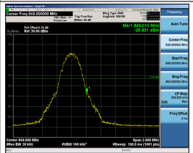
EGPRS850-251-8
