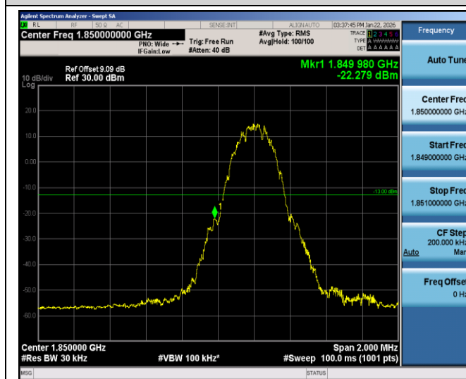
GSM1900-512-0
