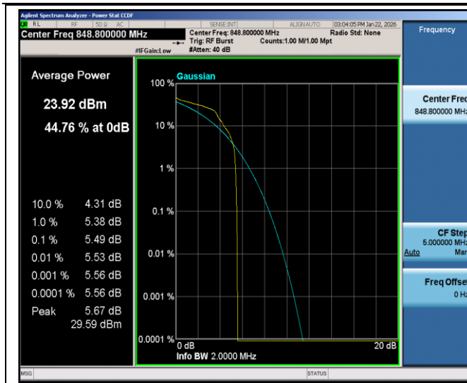
EGPRS850-251-8
