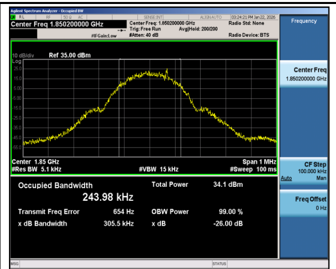
GSM1900-512-0-0.3055
