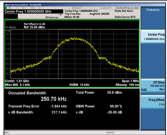
EGPRS1900-810-2-0.3171
