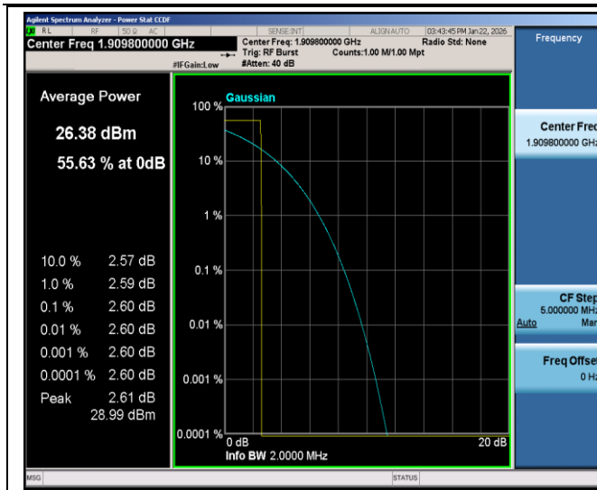
GPRS1900-810-0
