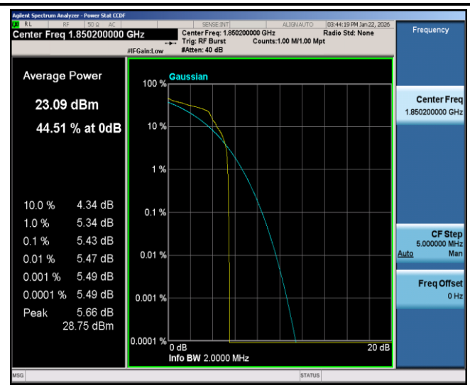
EGPRS1900-512-2
