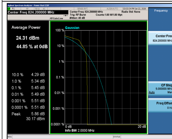
EGPRS850-128-8
