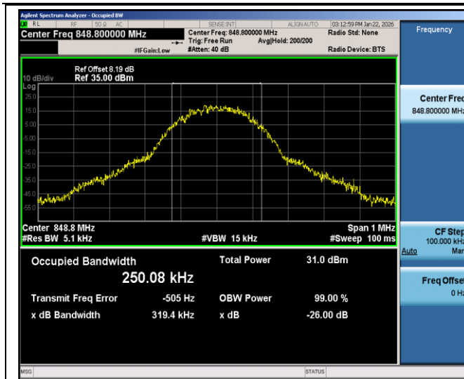
EGPRS850-251-8-0.3194
