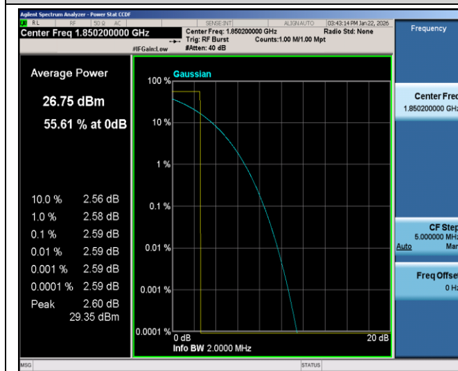
GPRS1900-512-0
