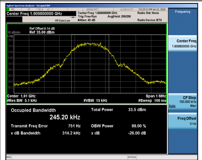
GSM1900-810-0-0.3142
