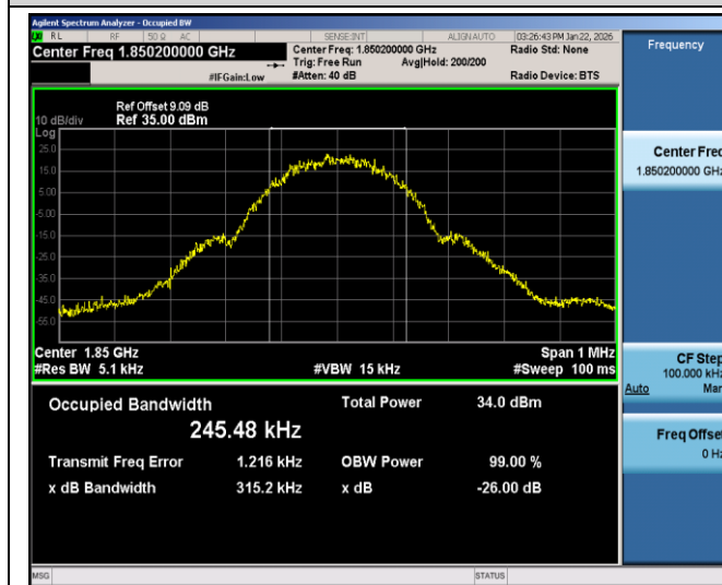
GPRS1900-512-0-0.3152
