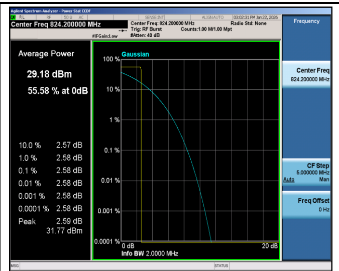
GPRS850-128-3
