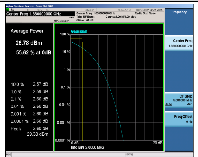
GPRS1900-661-0
