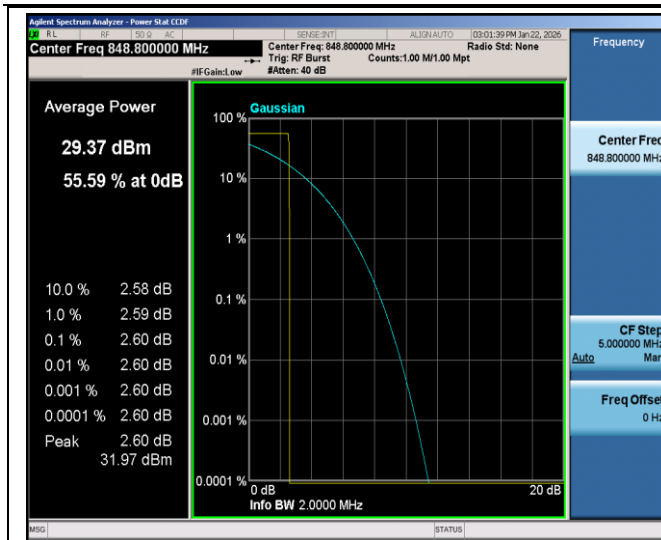
GSM850-251-3
