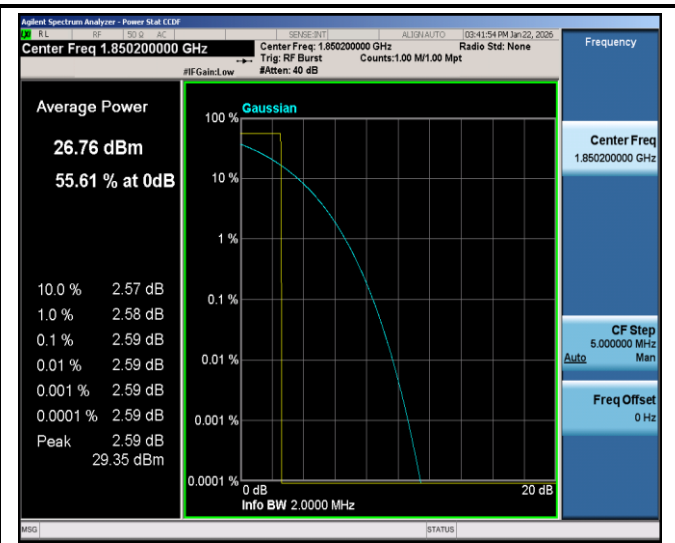
GSM1900-512-0
