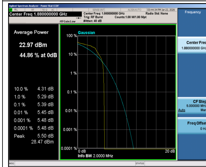
EGPRS1900-661-2
