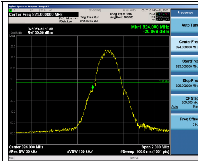
GPRS850-128-3
