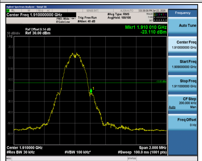
GSM1900-810-0
