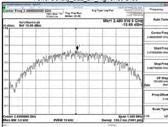
Power Density BLE 1M HighCH39-2480
