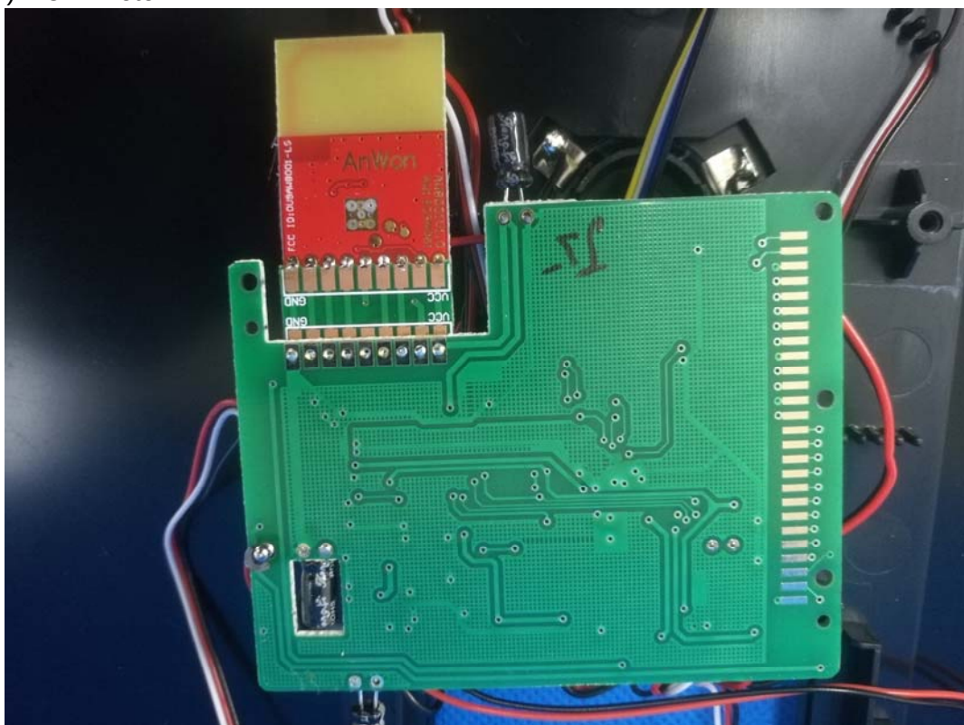
(4) EUT Photo
