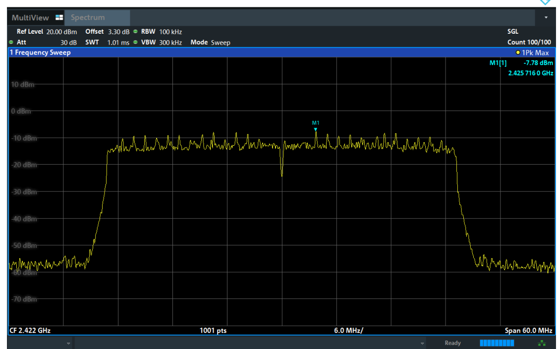
Band Edge NVNT ax40 2422MHz Ant1 Emission
