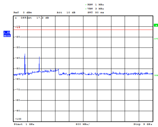
WCDMA Band V CH-Low 1GHz ~ 9GHz
