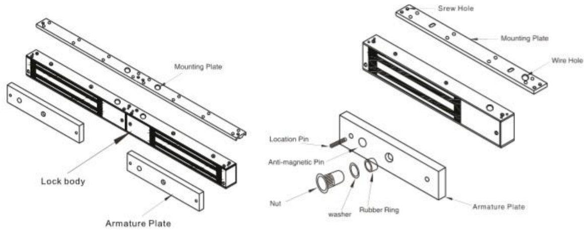
Double Door
