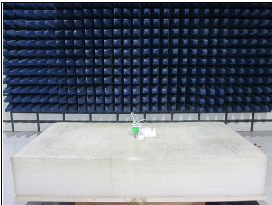
Z-plane (EUT) Mode A1
