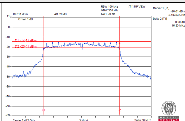
802.11g : CH 1
