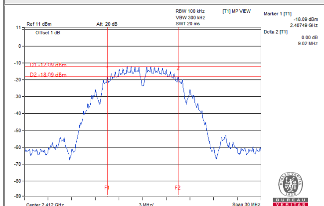
802.11b : CH 1
