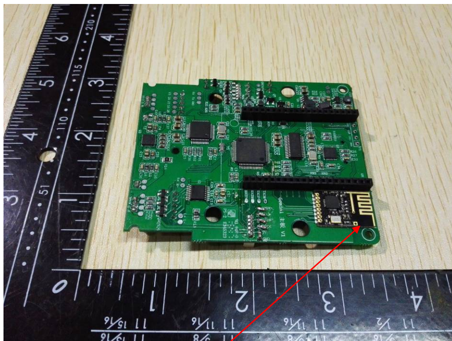
2.4G Module Antenna
