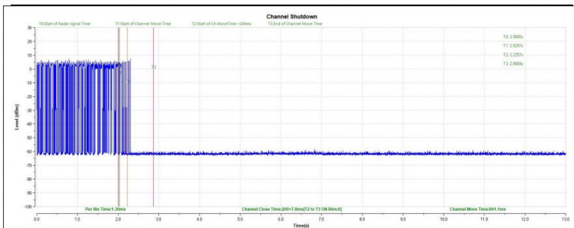
11AX80SISO-5290-Type0-PASS
