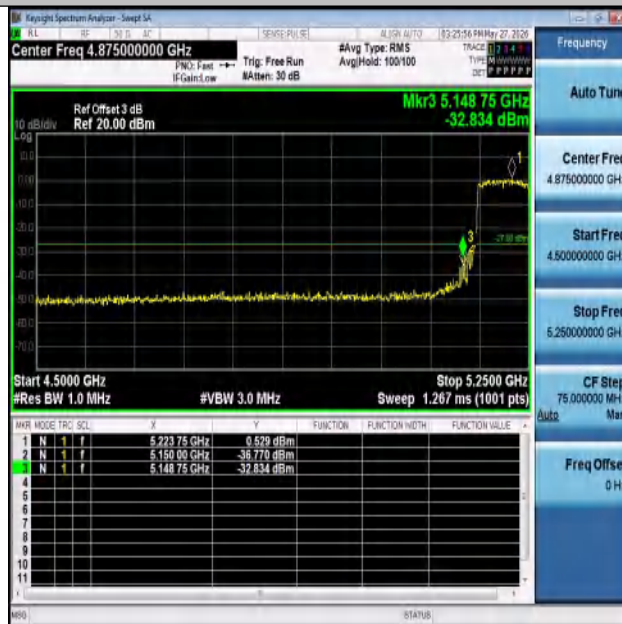
11AX80SISO-Ant1-5210-PASS
