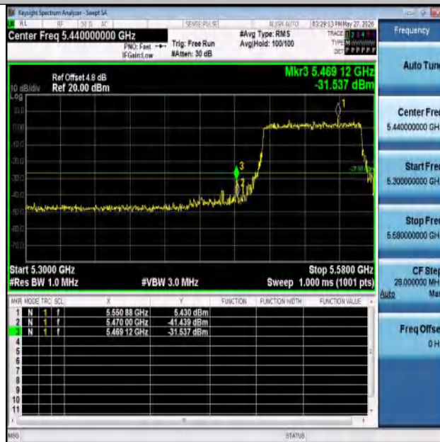
11AX80SISO-Ant1-5530-PASS
