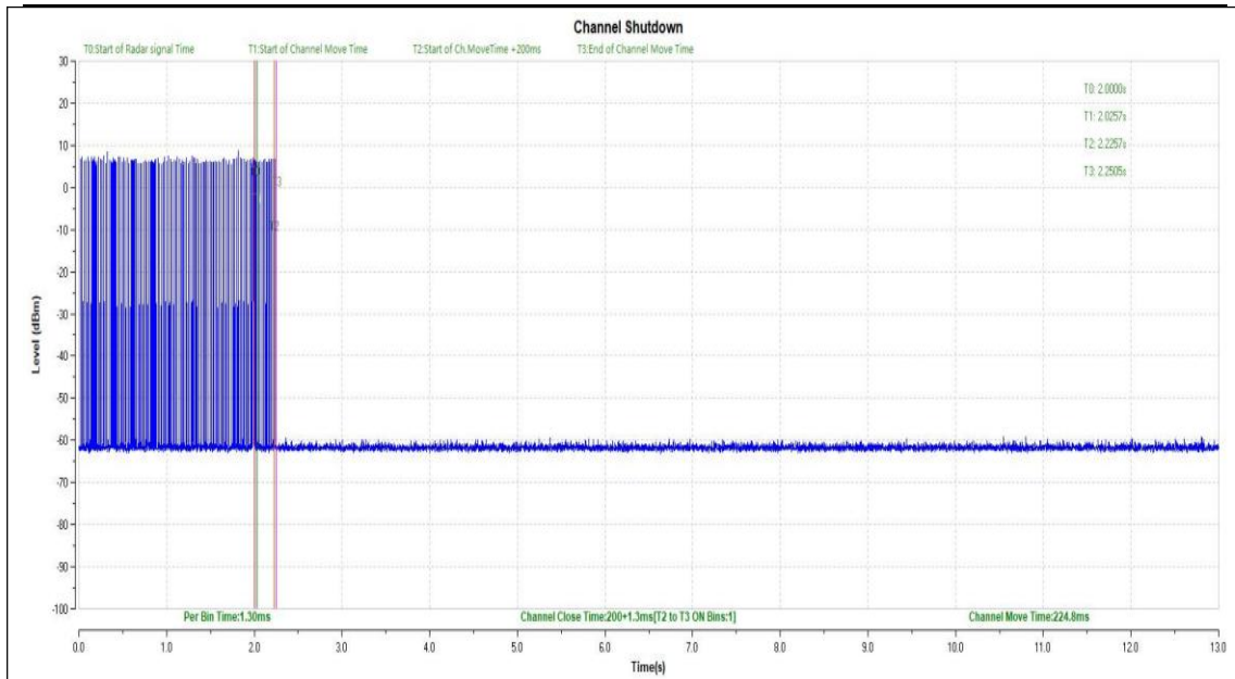
11AX80SISO-5290-Type0-PASS
