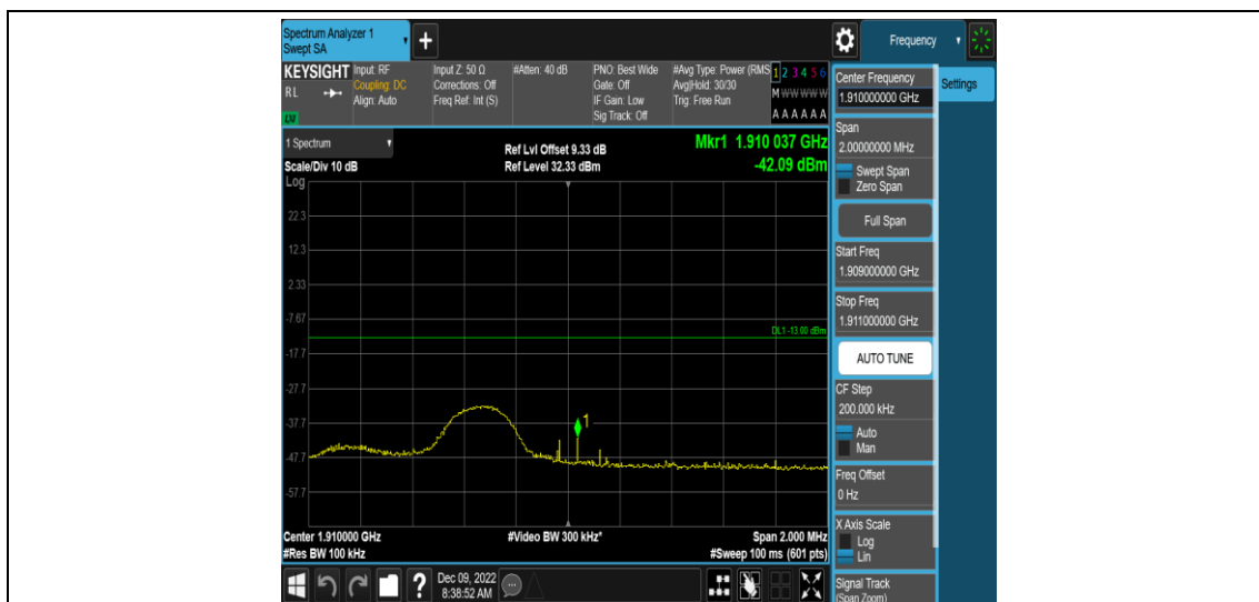
Band2-5MHz-QPSK-19175-1RB#24
