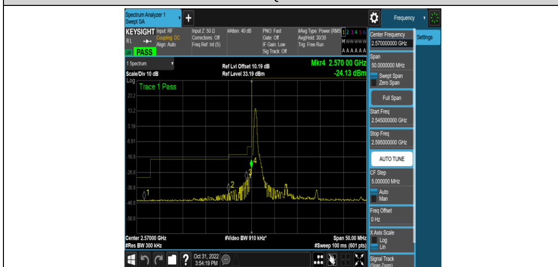
Band38-15MHz-QPSK-37825-1RB#74
