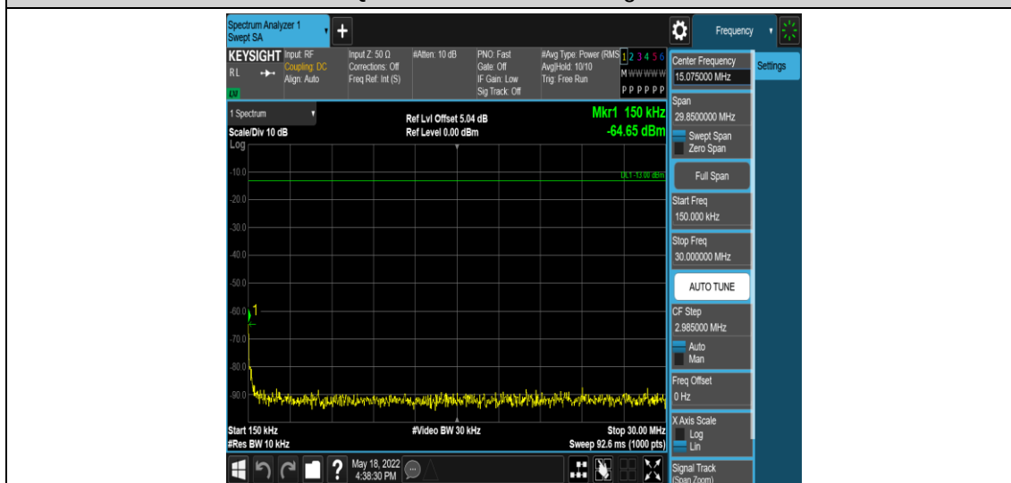
Band12-3MHz-QPSK-23095-1RB#0-Range2:0.15~30MHz
